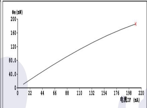
电流与光功率
