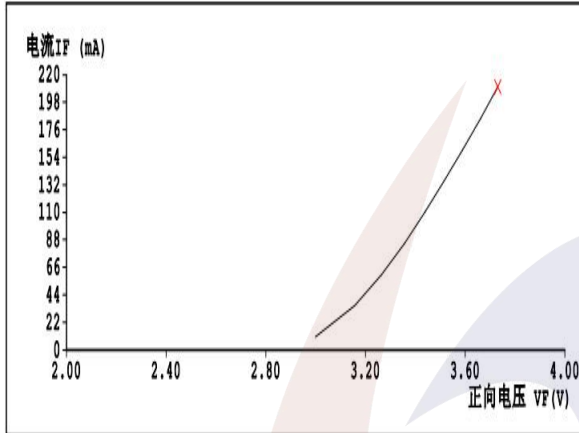
电压与电流
