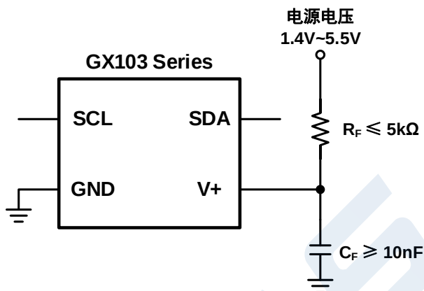
图 9 噪声消除技术
