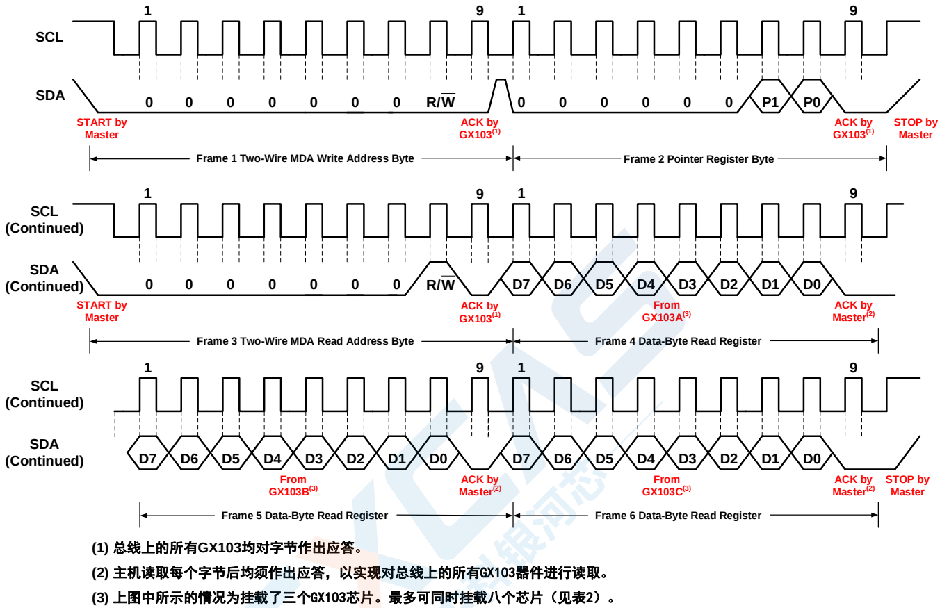
图 7 两线制 MDA 读命令时序图
