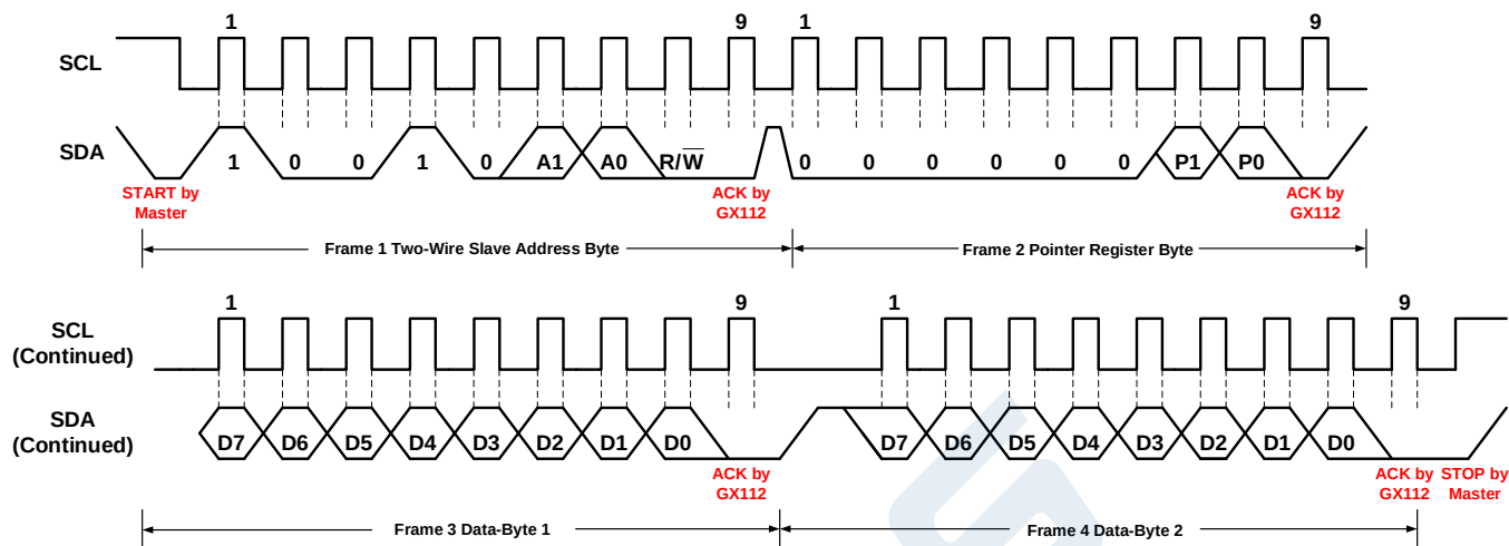
图 6 两线制写命令时序图
