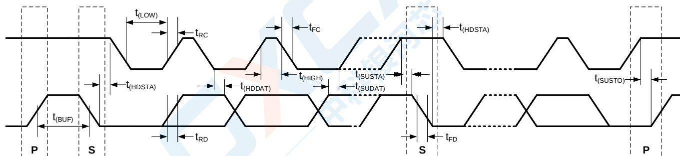
图 1 两线时序图
