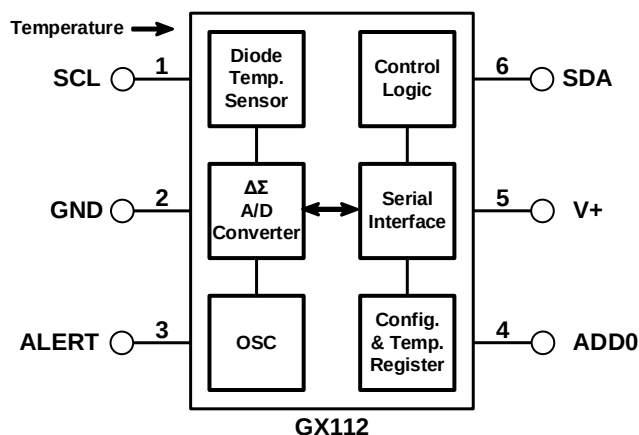
GX112 各模块示意图（SOT563 封装）
