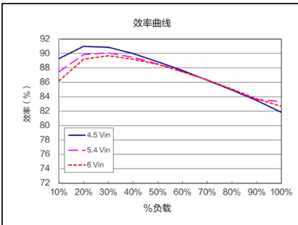
效率曲线 ( V_{nom}=5.4V , V_{out}=0.9V )
