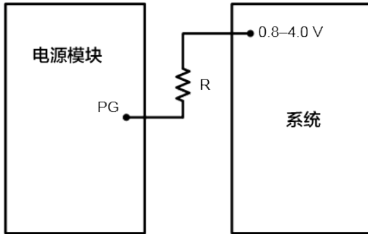
图 5-7 PG 配置图
