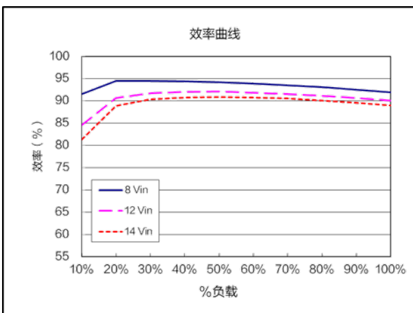
效率曲线 ( V_{nom}=12.0V , V_{out}=3.7V )
