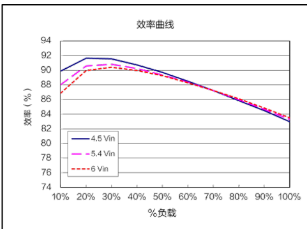
效率曲线 ( V_{nom}=5.4V , V_{out}=1.0V )
