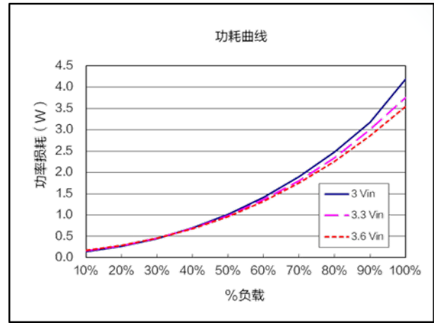
功耗曲线 ( V_{nom}=3.3V, V_{out}=0.8V )
