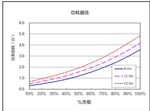
功耗曲线 ( V_{nom}=12.0V , V_{out}=0.6V )
