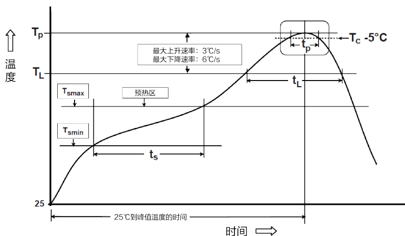
图 9-1 推荐无铅焊料回流曲线
