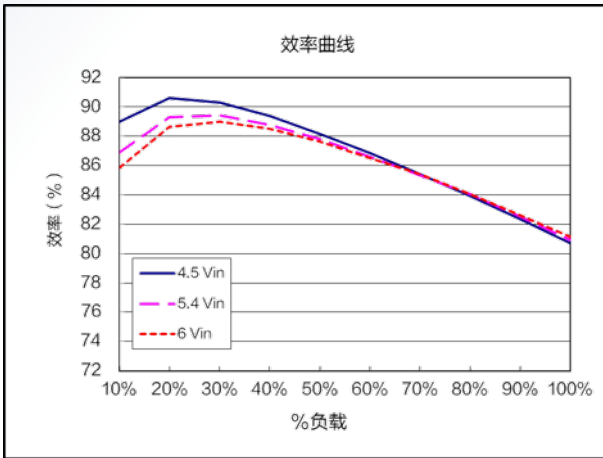
效率曲线 ( V_{nom}=5.4V , V_{out}=0.8V )
