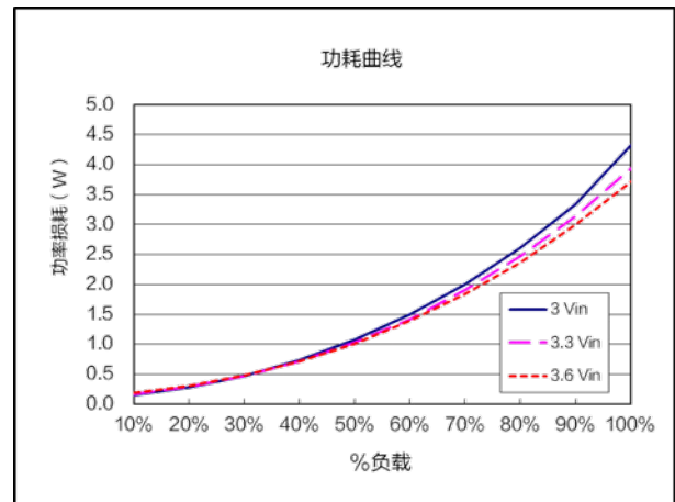
功耗曲线 ( V_{nom}=3.3V, V_{out}=0.9V )
