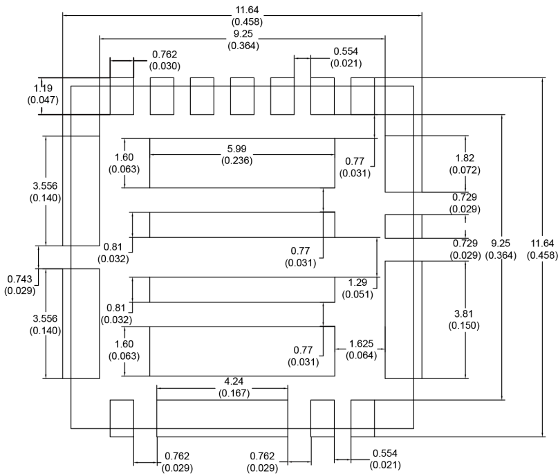
图 5-1 封装尺寸图
