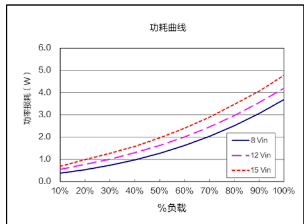
功耗曲线 ( V_{nom}=12.0V , V_{out}=1.0V )
