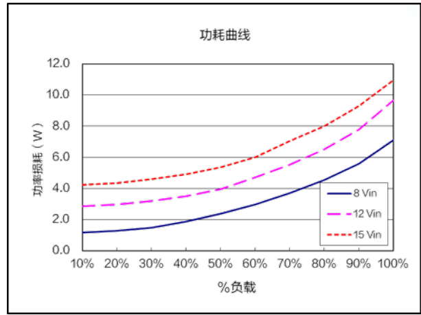
功耗曲线 ( V_{nom}=12.0V , V_{out}=5.0V )
