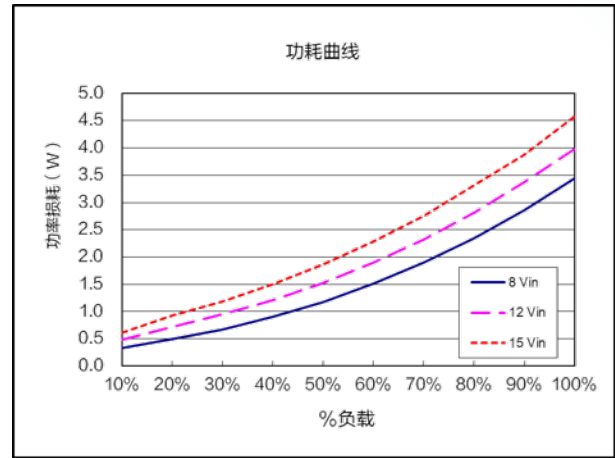
功耗曲线 ( V_{nom}=12.0V , V_{out}=0.8V )
