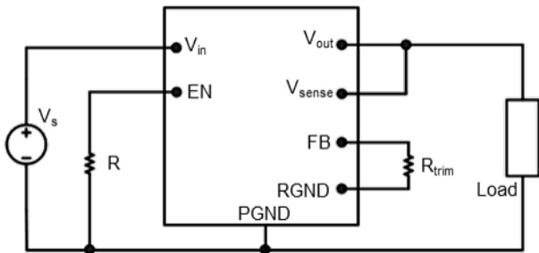
图 5-5 EN 功能电路配置图
