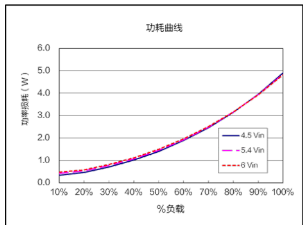
功耗曲线 ( V_{nom}=5.4V , V_{out}=1.8V )
