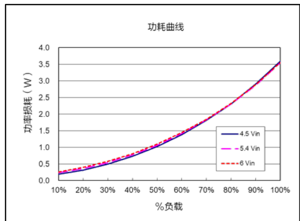
功耗曲线 ( V_{nom}=5.4V , V_{out}=0.7V )
