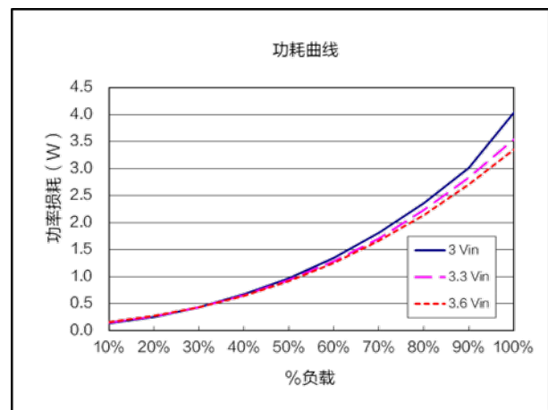
功耗曲线 ( V_{nom}=3.3V, V_{out}=0.7V )
