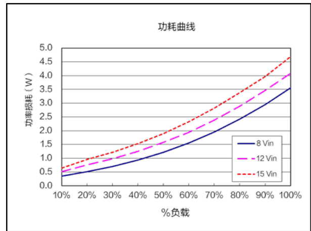
功耗曲线 ( V_{nom}=12.0V , V_{out}=0.9V )
