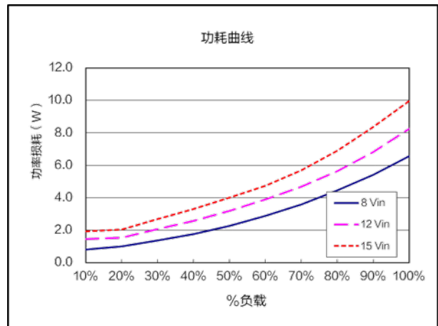
功耗曲线 ( V_{nom}=12.0V , V_{out}=3.3V )
