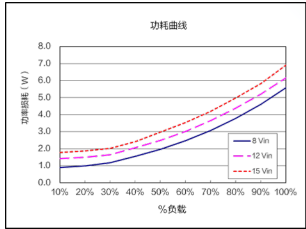
功耗曲线 ( V_{nom}=12.0V , V_{out}=2.5V )
