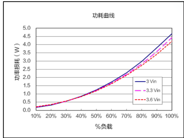
功耗曲线 ( V_{nom}=3.3V , V_{out}=1.2V )
