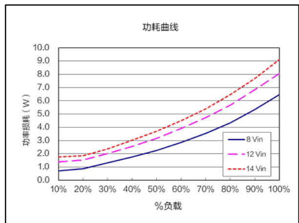
功耗曲线 ( V_{nom}=12.0V , V_{out}=3.7V )
