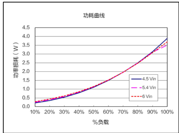
功耗曲线 ( V_{nom}=5.4V , V_{out}=0.9V )
