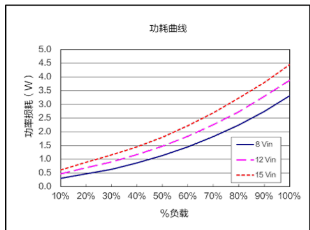
功耗曲线 ( V_{nom}=12.0V , V_{out}=0.7V )
