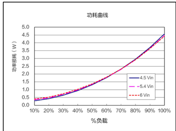
功耗曲线 ( V_{nom}=5.4V , V_{out}=1.5V )
