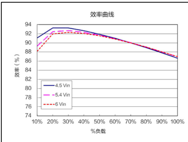
效率曲线 ( V_{nom}=5.4V , V_{out}=1.5V )
