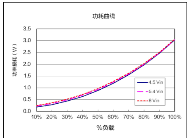
功耗曲线 ( V_{nom}=5.4V , V_{out}=0.6V )
