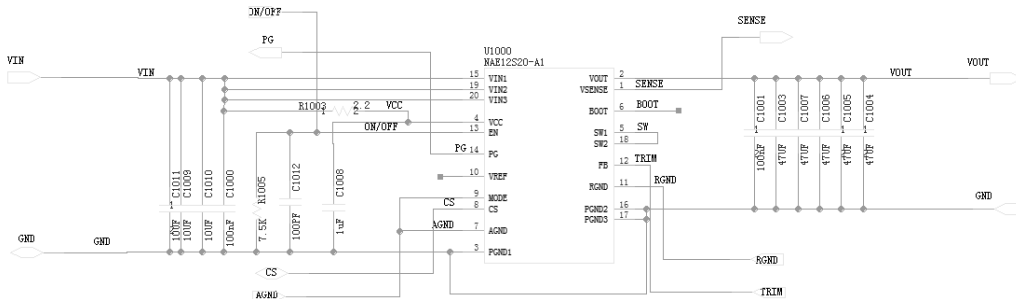
图 4-1 推荐应用电路
