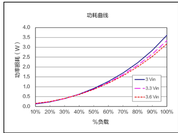
功耗曲线 ( V_{nom}=3.3V, V_{out}=0.6V )
