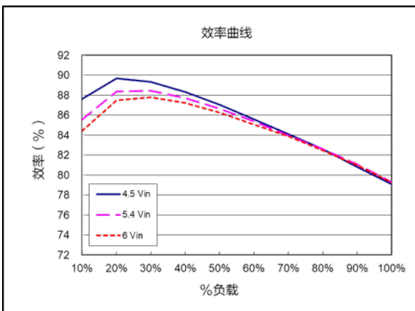
效率曲线 ( V_{nom}=5.4V , V_{out}=0.7V )
