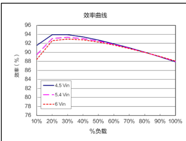
效率曲线 ( V_{nom}=5.4V , V_{out}=1.8V )
