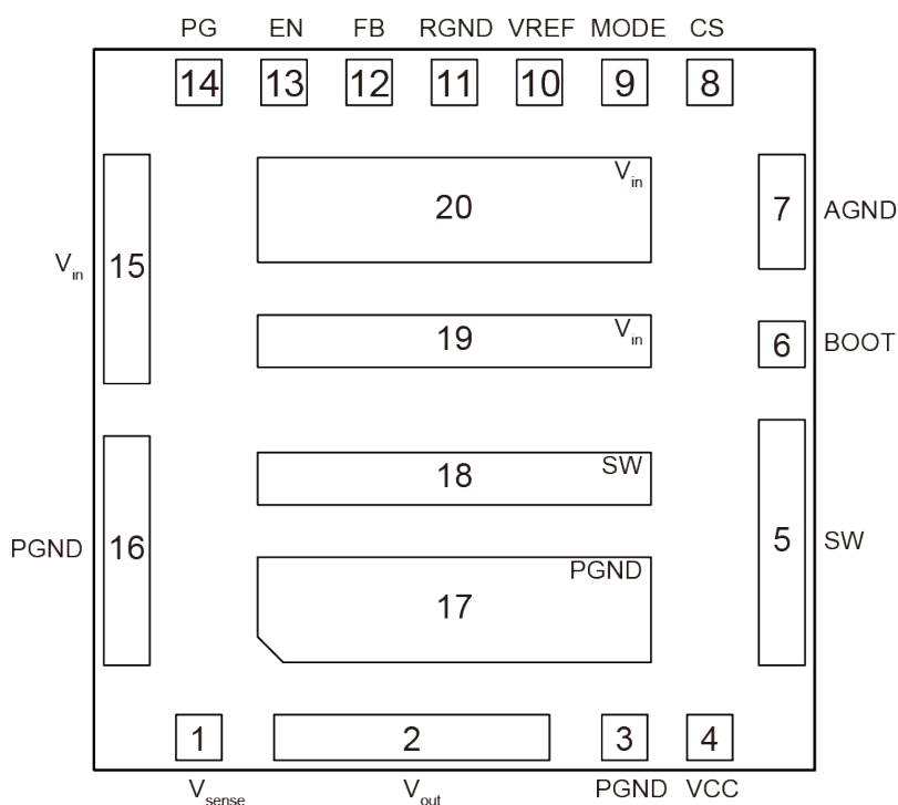
图 5-3 引脚分布
