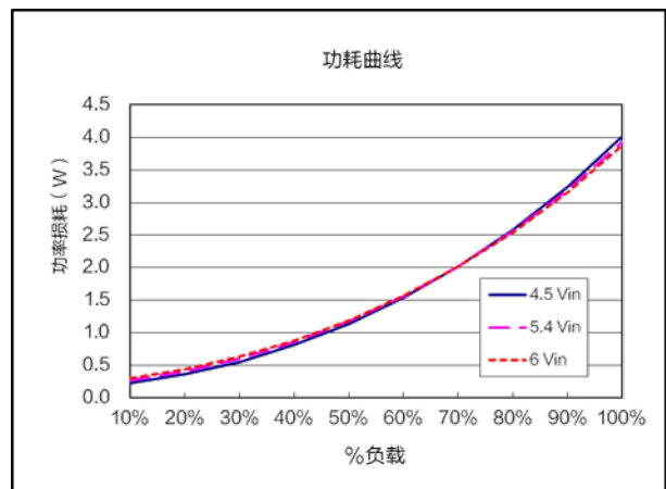
功耗曲线 ( V_{nom}=5.4V , V_{out}=1.0V )
