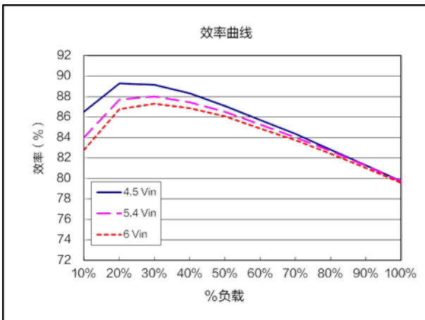
效率曲线 ( V_{nom}=5.4V , V_{out}=0.6V )
