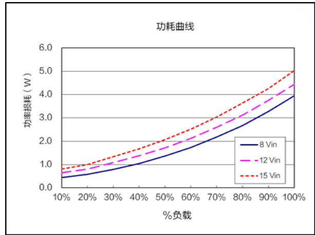
功耗曲线 ( V_{nom}=12.0V , V_{out}=1.2V )
