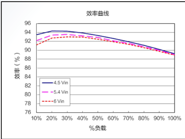
效率曲线 ( V_{nom}=5.4V , V_{out}=2.1V )
