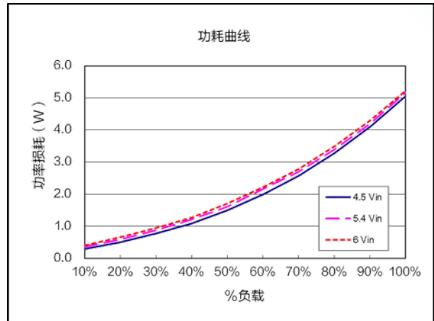
功耗曲线 ( V_{nom}=5.4V , V_{out}=2.1V )
