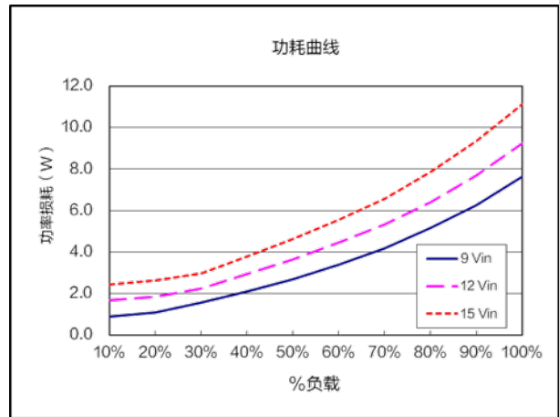
功耗曲线 ( V_{nom}=12.0V , V_{out}=5.5V )
