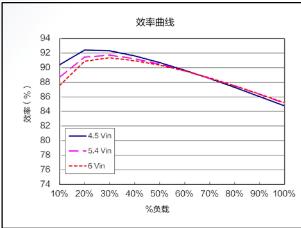
效率曲线 ( V_{nom}=5.4V , V_{out}=1.2V )
