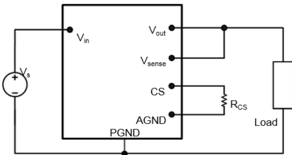
图 5-8 R CS 外部连接
