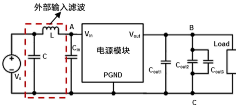
图 4-2 测试电路图
