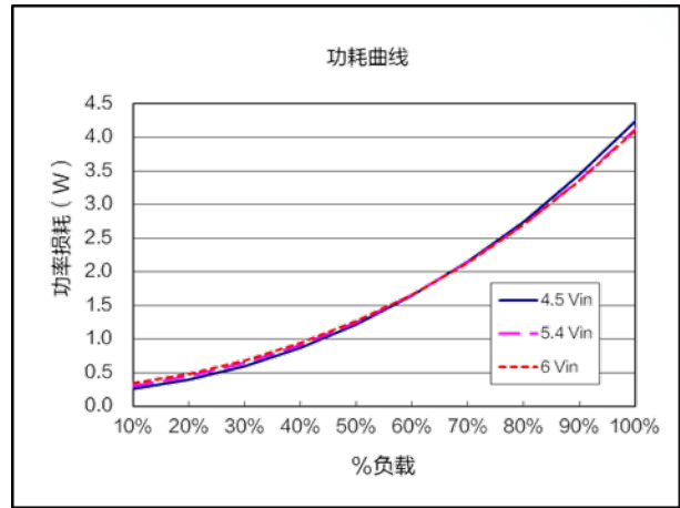
功耗曲线 ( V_{nom}=5.4V , V_{out}=1.2V )
