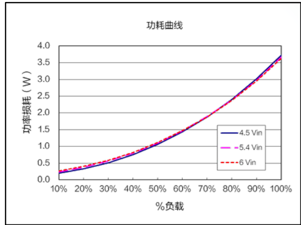
功耗曲线 ( V_{nom}=5.4V , V_{out}=0.8V )
