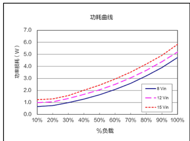
功耗曲线 ( V_{nom}=12.0V , V_{out}=1.8V )
