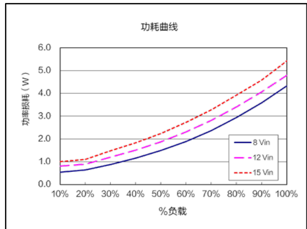
功耗曲线 ( V_{nom}=12.0V , V_{out}=1.5V )
