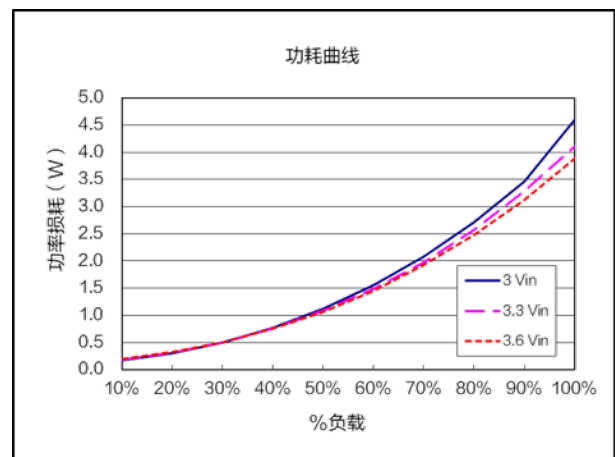
功耗曲线 ( V_{nom}=3.3V, V_{out}=1.0V )
