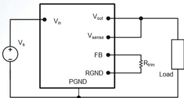
图 5-6 R trim 外部连接
