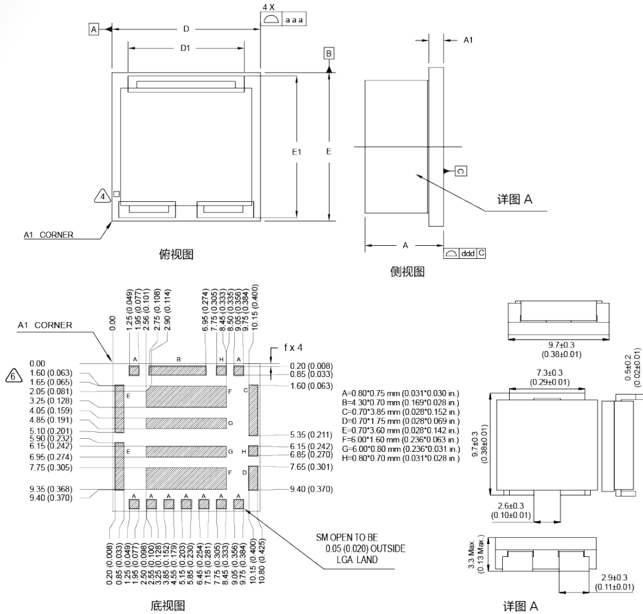
图 5-2 结构尺寸图
