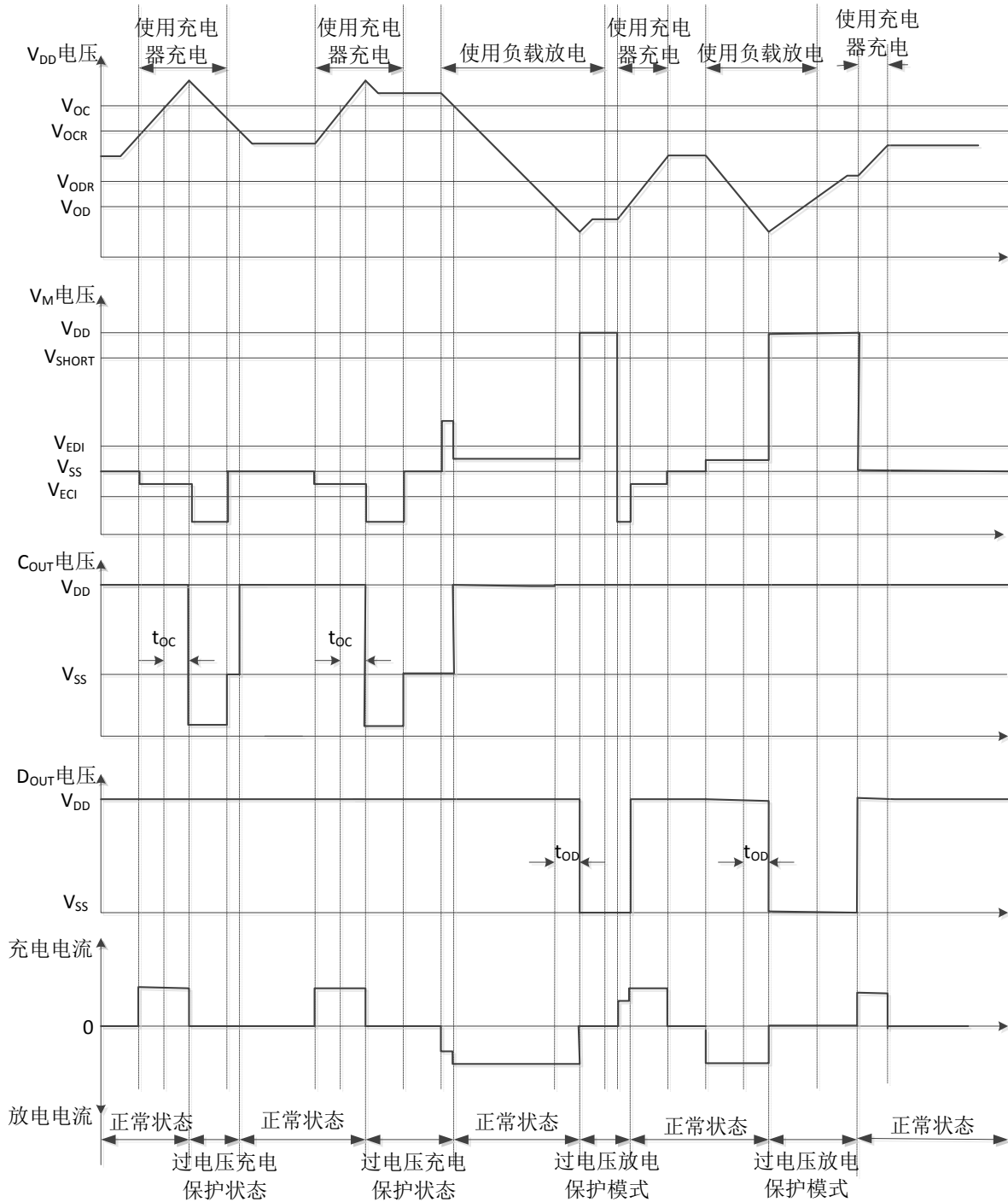
图-5 过电压充电和过电压放电保护状态各点波形图 (过放自恢复禁止型号)
