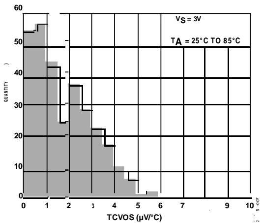
图7. 输入失调电压漂移分布图
