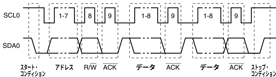
図18-12 I 2 Cバスのシリアル・データ転送タイミング
