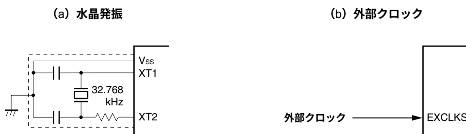
図6-13 XT1発振回路の外付け回路例
