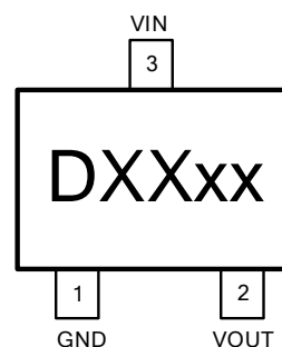
SOT23
