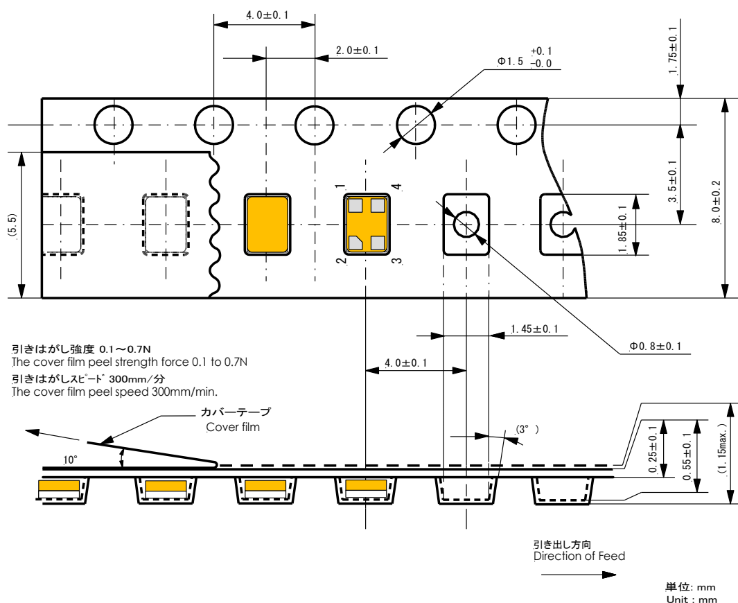
第2図 プラスチックテープの外形寸法図
