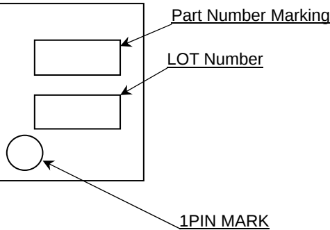
SSOP-B14(TOP VIEW)
