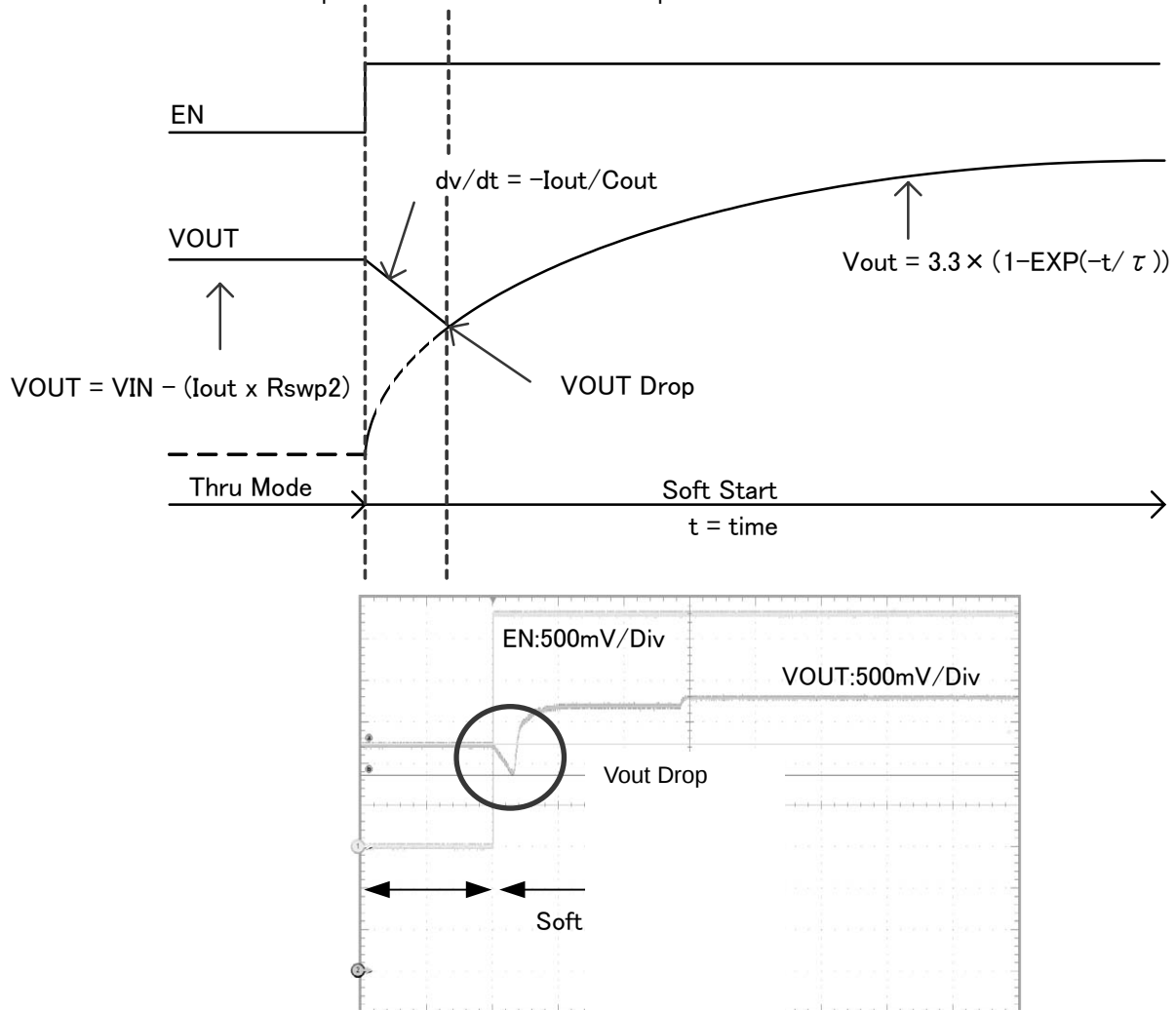
Figure 47. EN : L=>H PFM I_o=5\text{mA} VIN=3.6V
