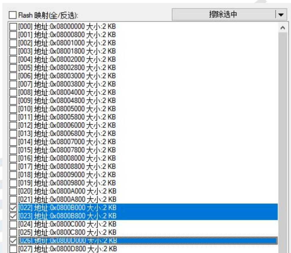
图 3.1.4.3-6 Power Writer 扇区表
