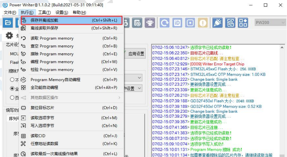
图 4.2.2-4 将项目保存到本地并离线加载到 Power Writer
