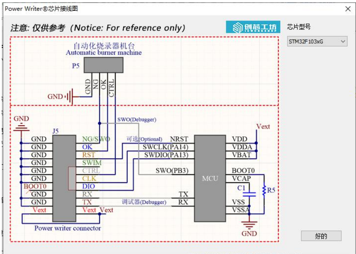
图 3.1.2.3.3 Power Writer 快速查询芯片接线图
