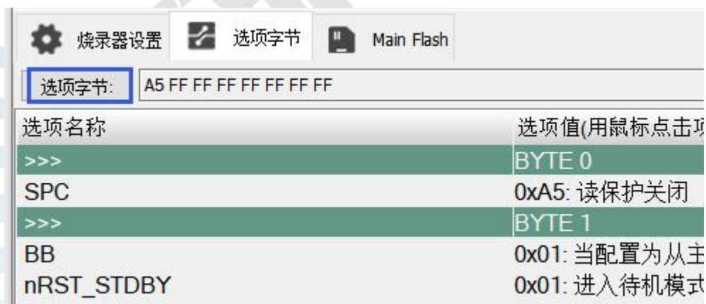
图 3.1.4.2-3 选项字节缓冲区编辑入口
