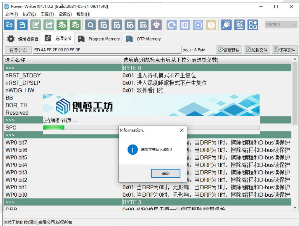
图 4.1.2 -2 Power Writer 在线更新选项字节
