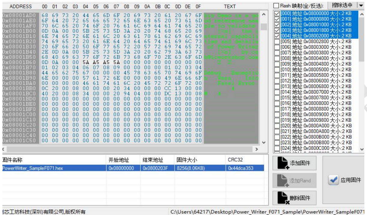
图 4.2.2-3 添加编译出的固件到 Power Writer 的 Program Memory
