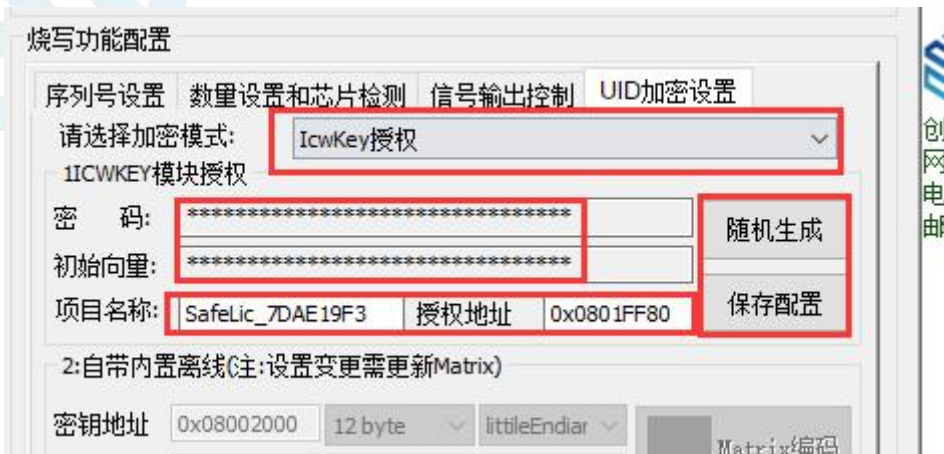
图 4.2.4-3 Power Writer ICWKEY 授权方式设置界面
