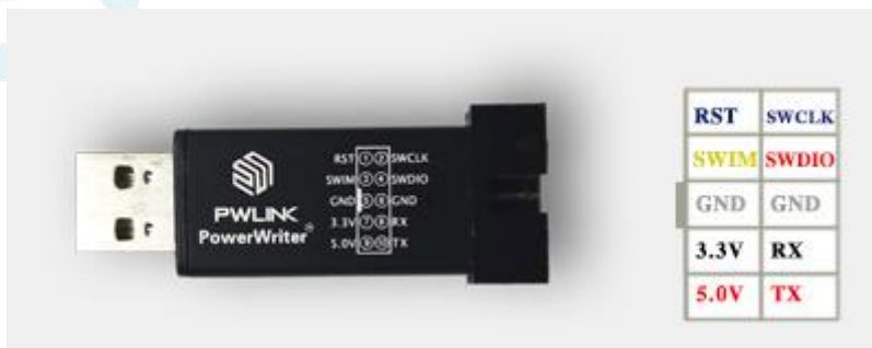
图 2.3.2-b Power Writer For ARM Link (PWLINK)外观
