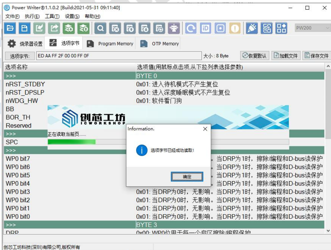
图 4.1.2 -1 Power Writer 在线读取选项字节
