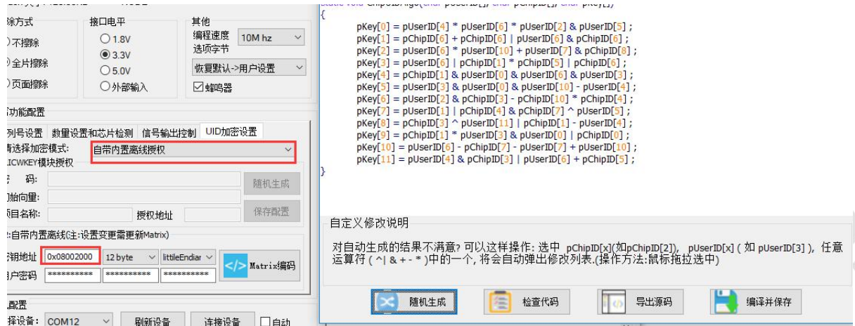
图 4.2.2-3 Power Writer 设置第四页
