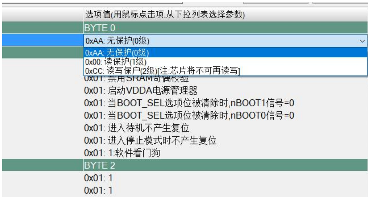
图 3.1.4.2-2 选项字节更改方法
