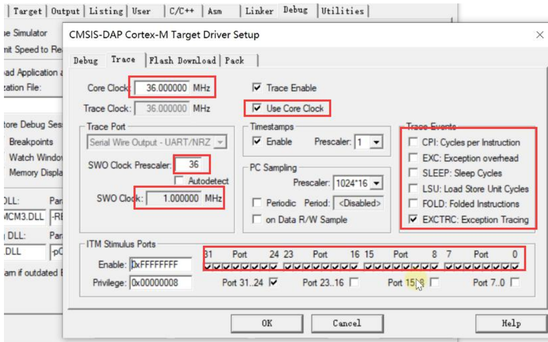
图 4.1.1.3-2 MDK 中开启 ITM Trace 功能
