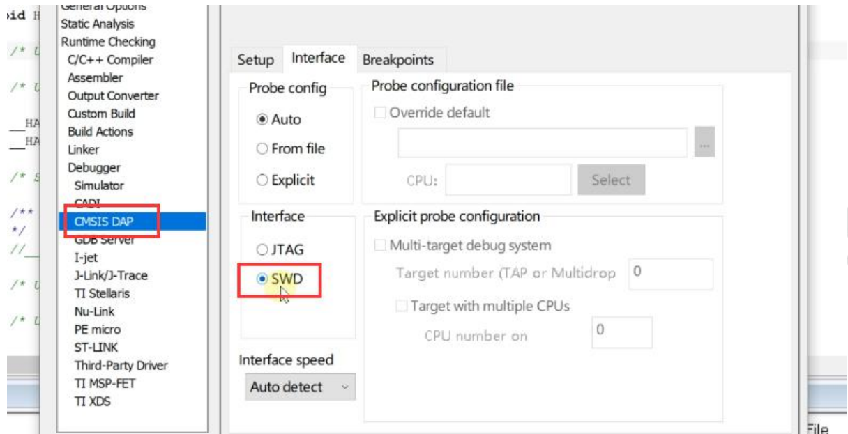
图 4.1.1.4-2 Power Writer IAR 调试器接口设置
