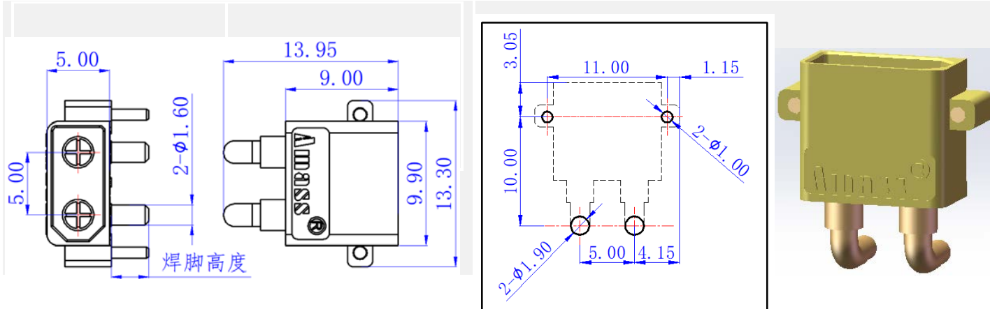
安装孔示意图
