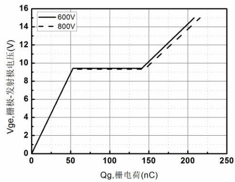
图 6 栅电荷特性
