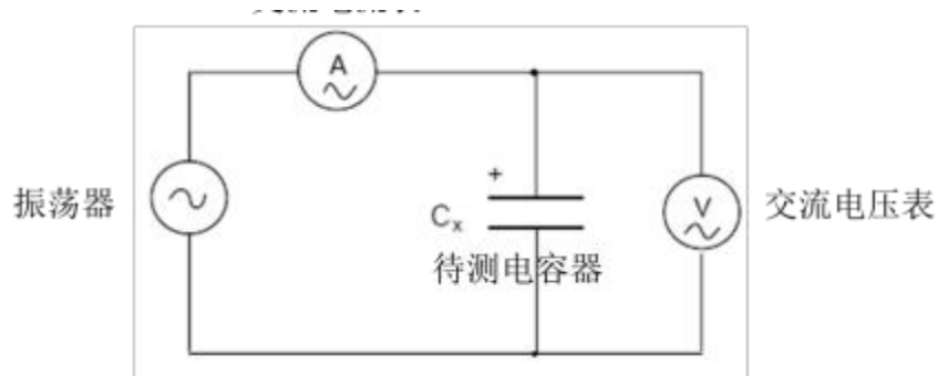
图 3 交流内阻测试电路
