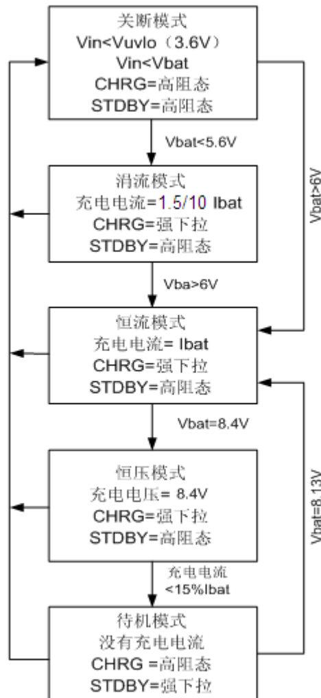
图 1: 一个典型的充电循环状态图
