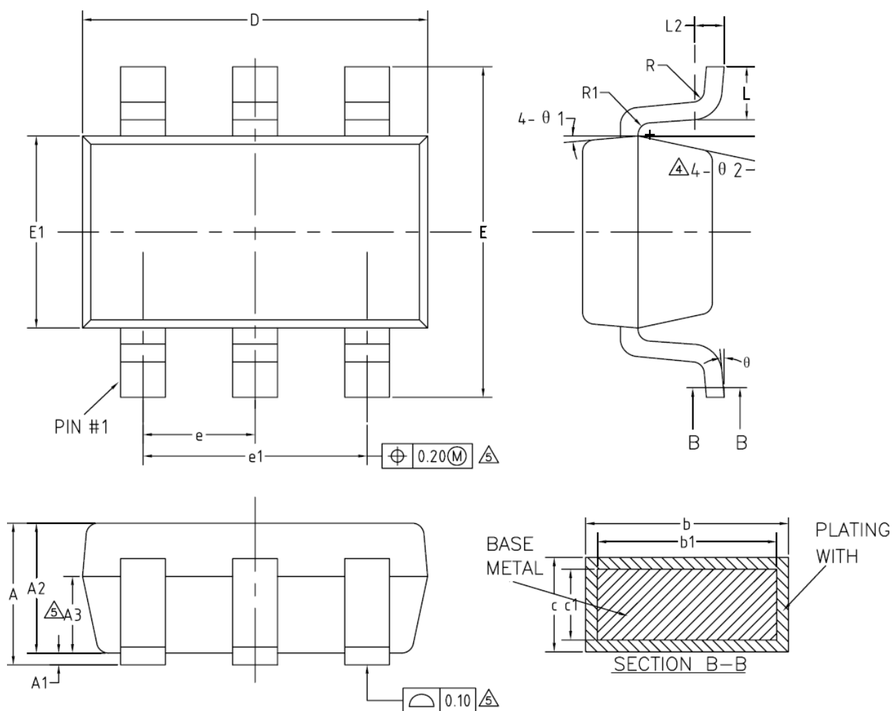
图 2 SOT23-6 封装
