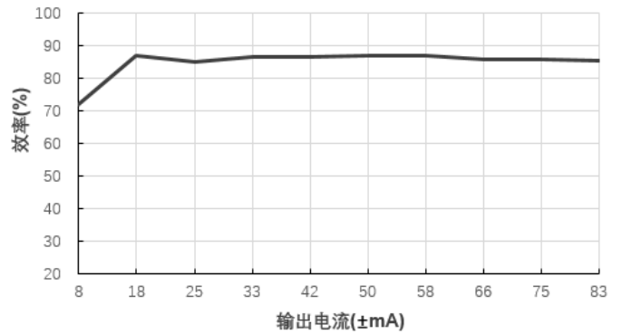
效率Vs输出电流( V_{in}=12V )@E1205S-2WR3
