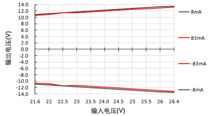
输出电压Vs输入电压@E2412S-2WR3
