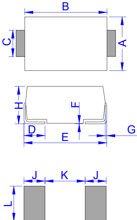
DO-214AC (SMA)
