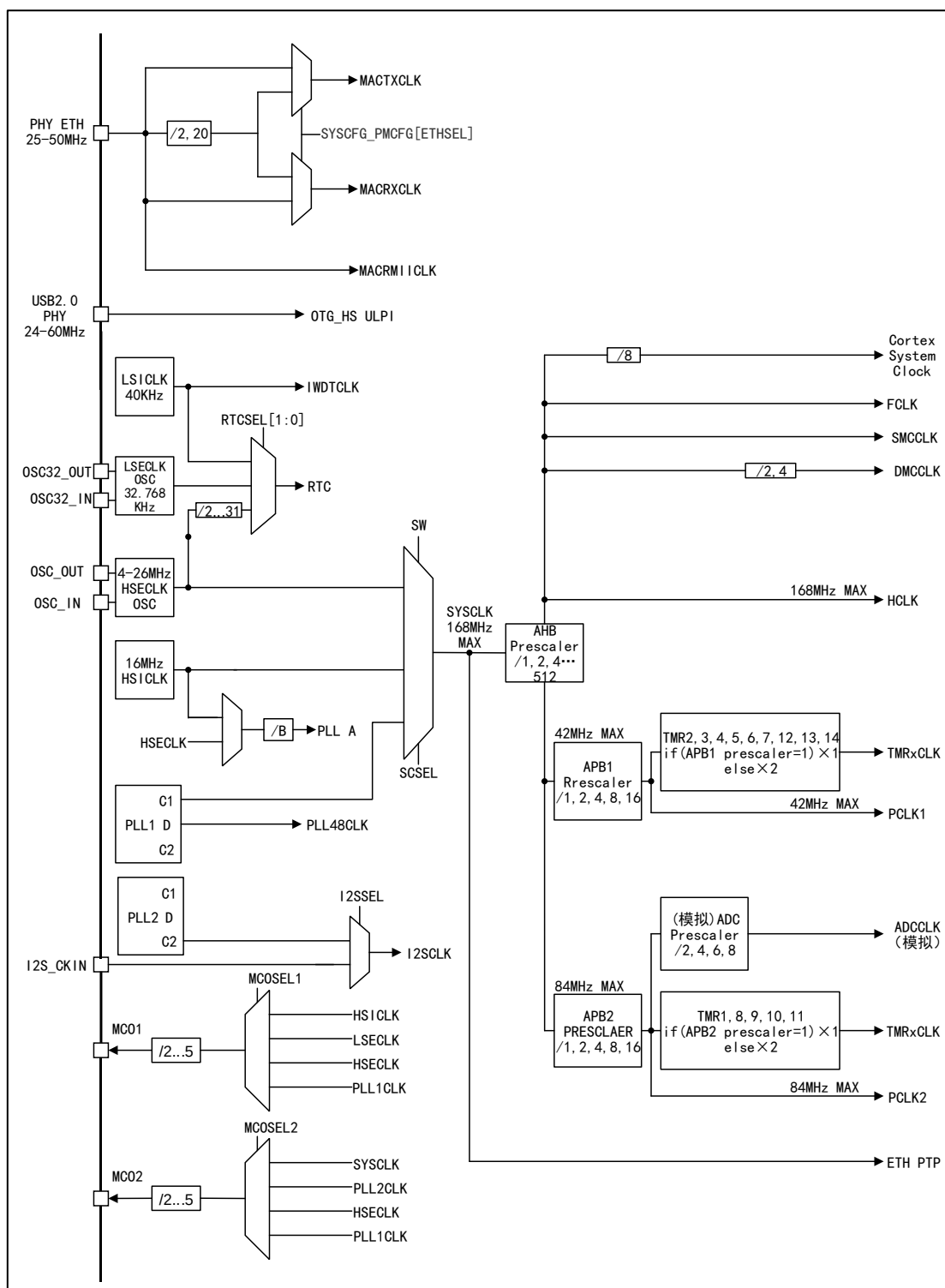
图 7 APM32F405xG 407xExG 时钟树
