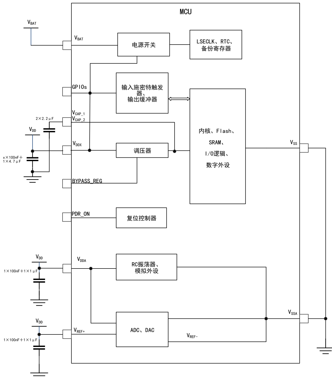
图 8 电源方案
