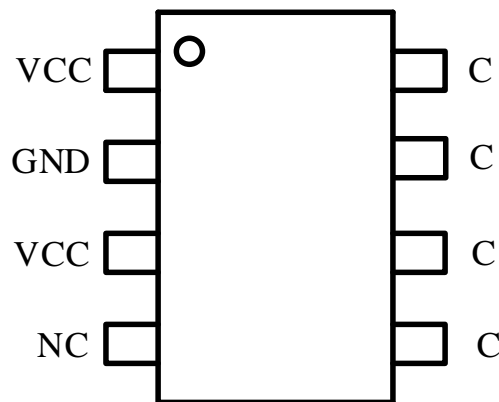
图 2 管脚封装图
