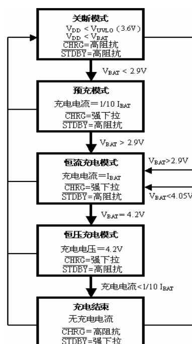
图 1：一个典型充电循环的状态图
