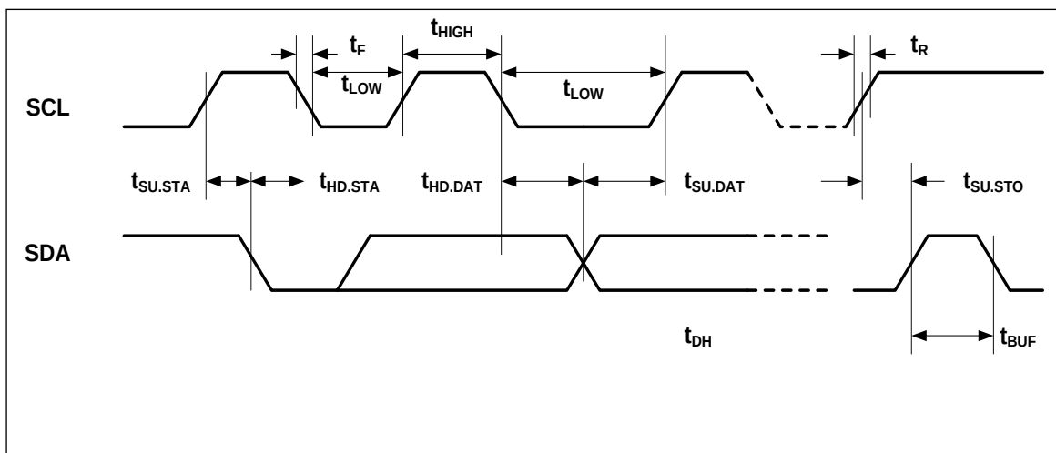
图 18-2 I²C 总线时序
