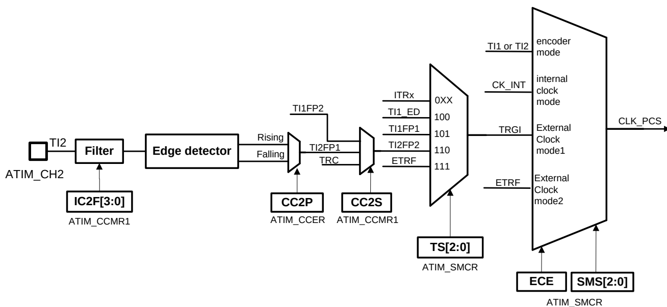
图 28-17 TI2 外部时钟连接例子
