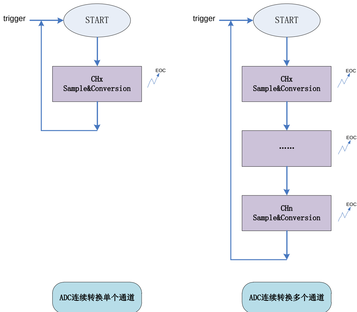
图 33-8 ADC 连续转换模式
