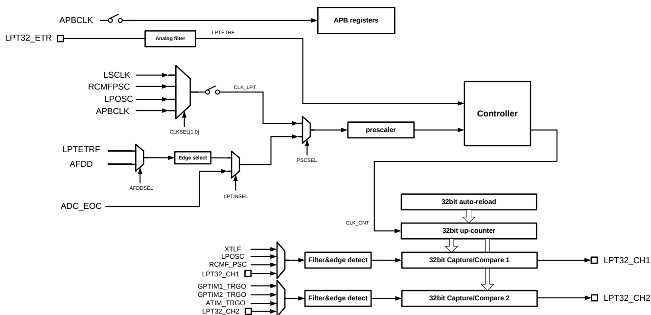
图 30-1LPTIM32 结构框图
