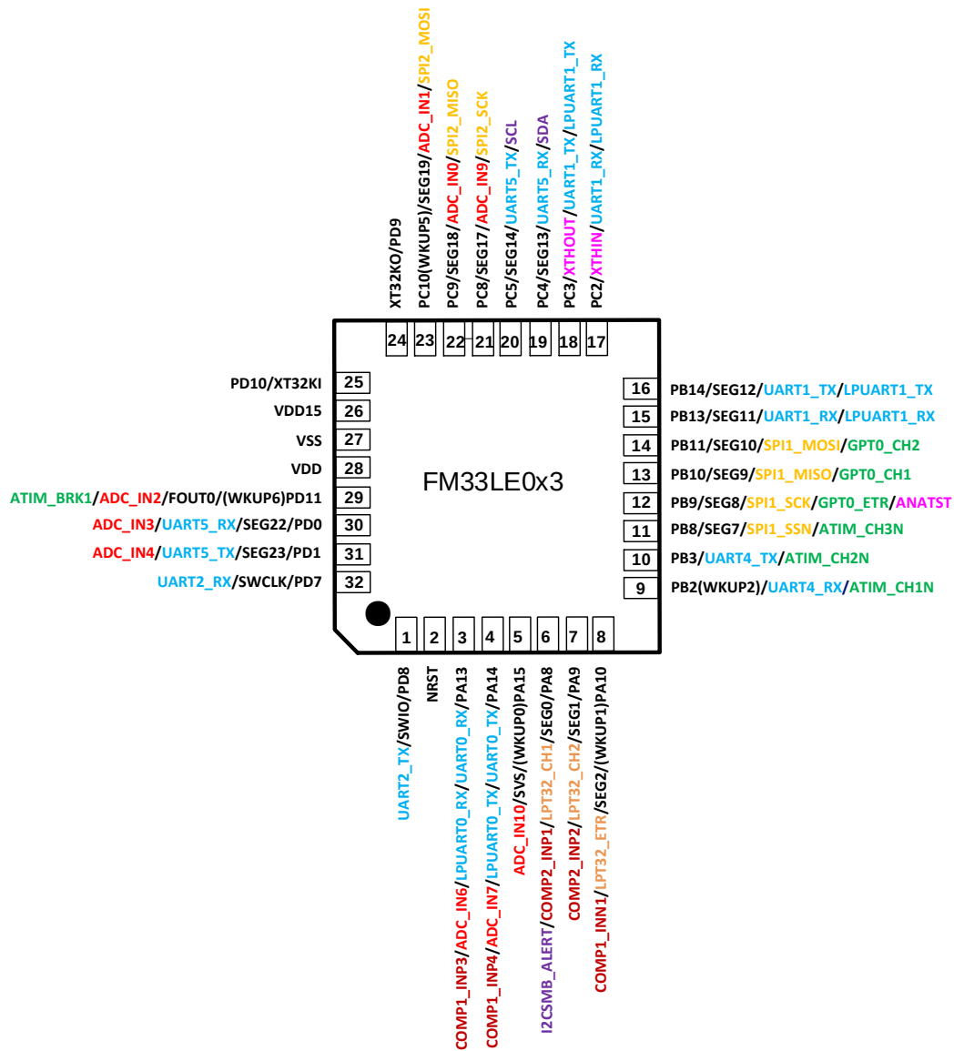
图 2-3FM33LE0x3QFN32 封装图
