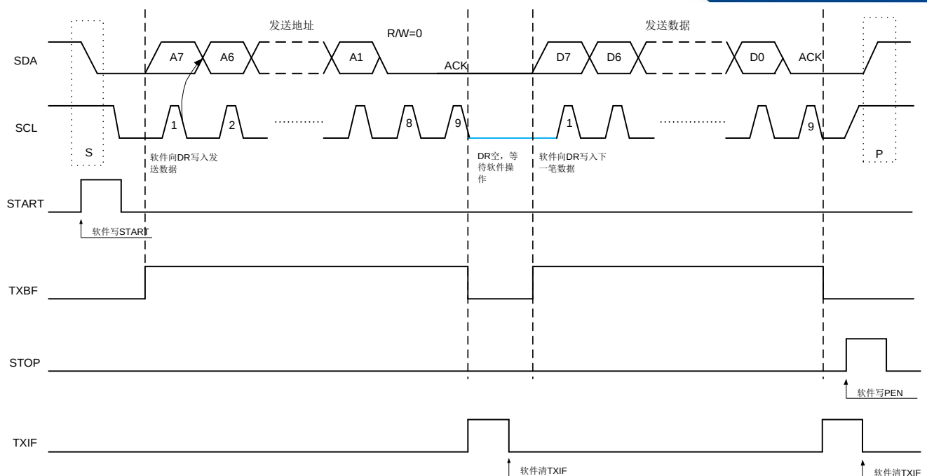
图 18-9 I²C 主机对 7 位地址从机发送数据流程图
