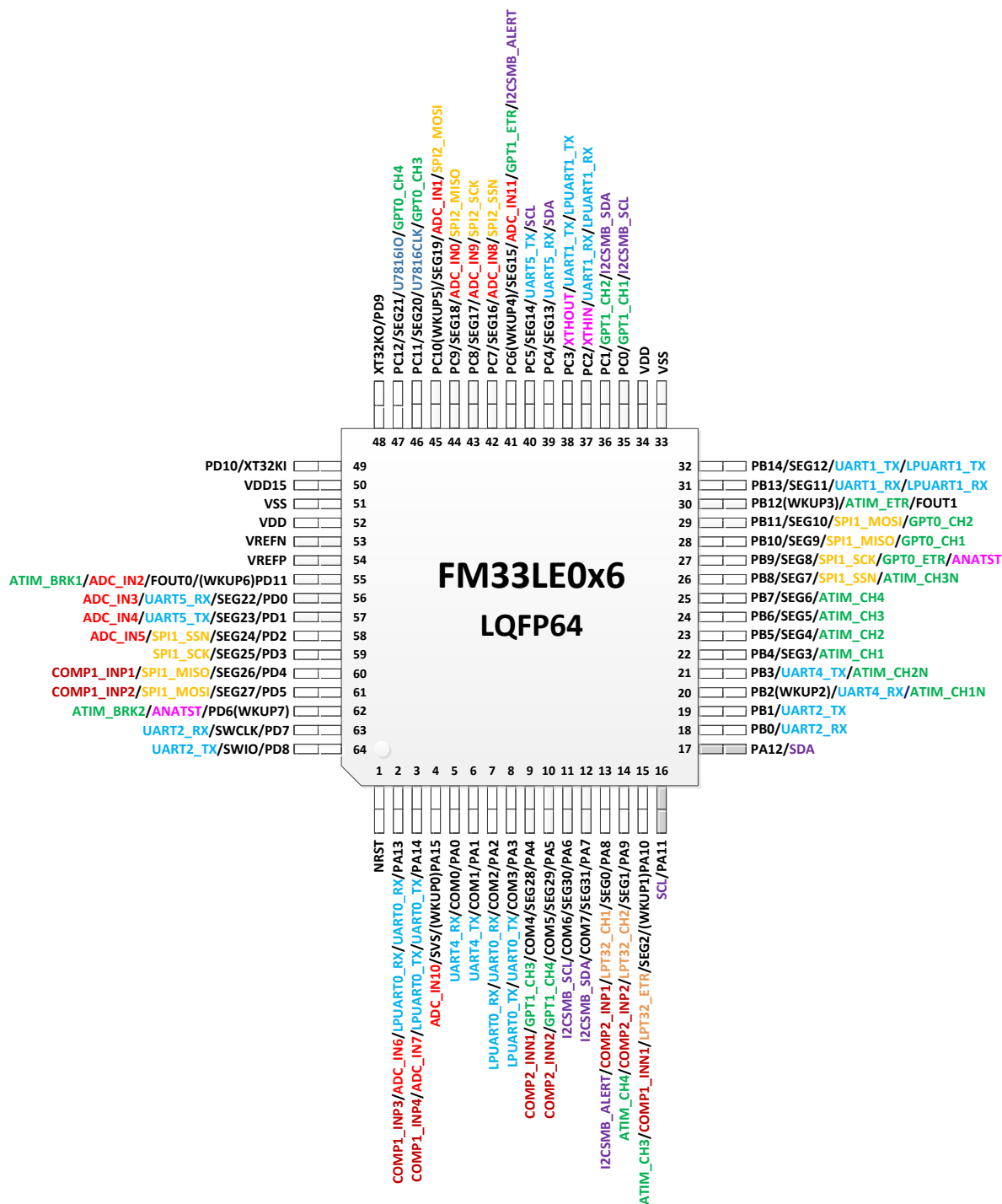
图 2-1FM33LE0x6 LQFP64 封装图
