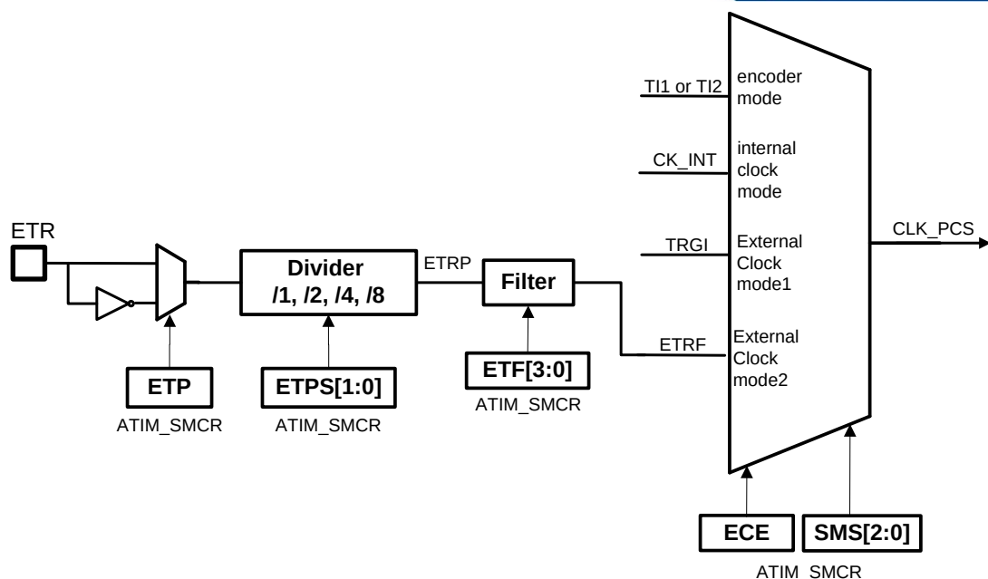
图 28-20 外部触发输入框图
