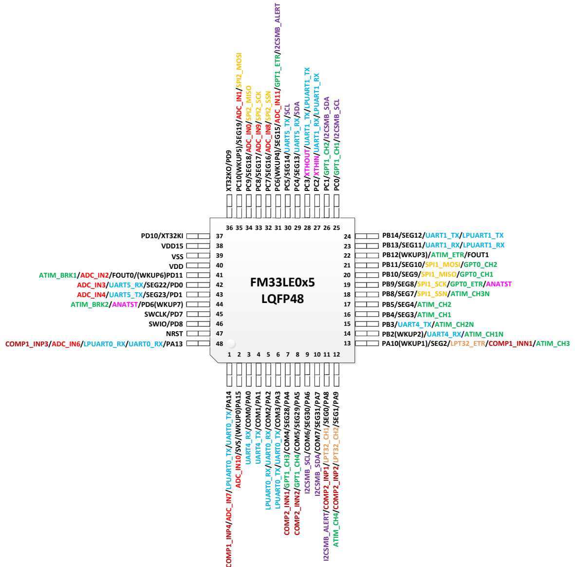
图 2-2FM33LE0x5 LQFP48 封装图
