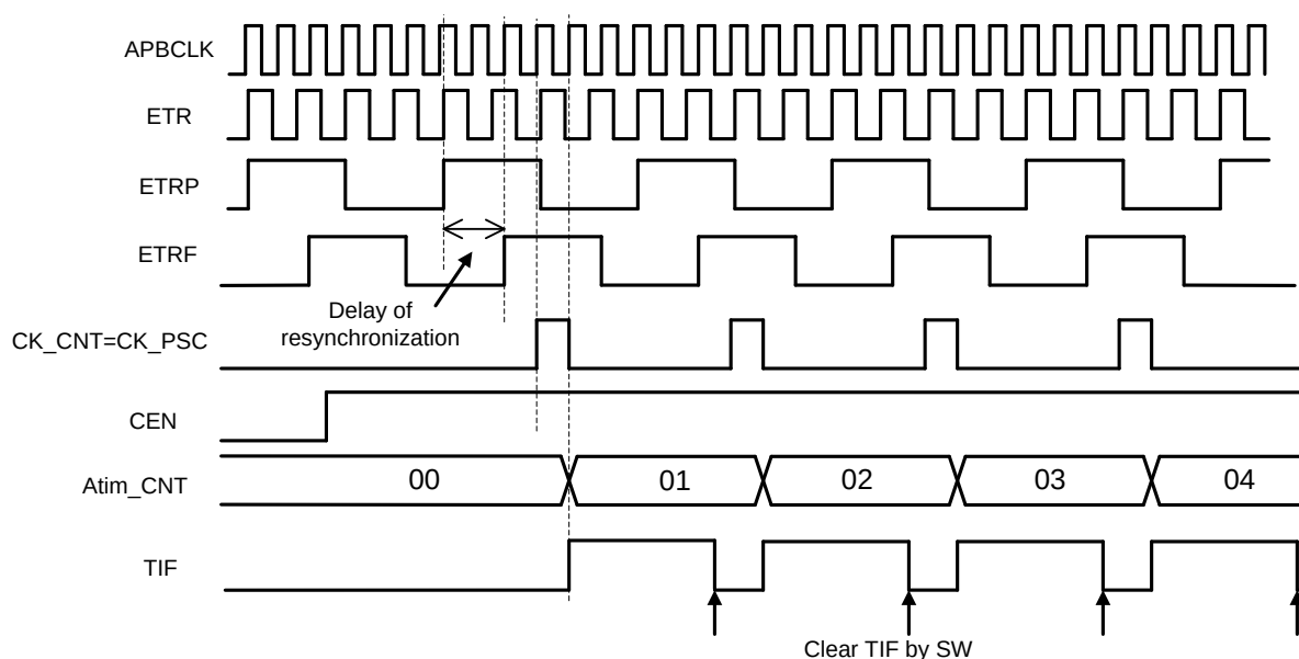
图28-22外部时钟模式2下的时序2
