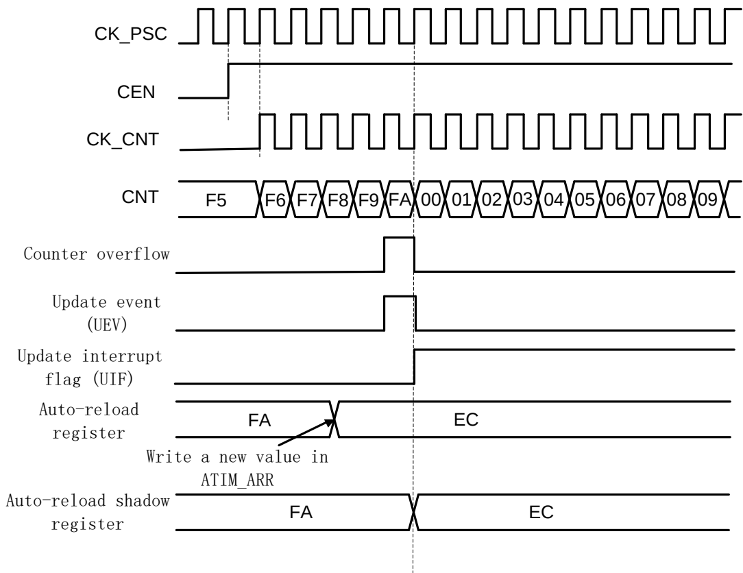
图 29-7 ARPE=1 (ARR 预装载) 时的更新事件
