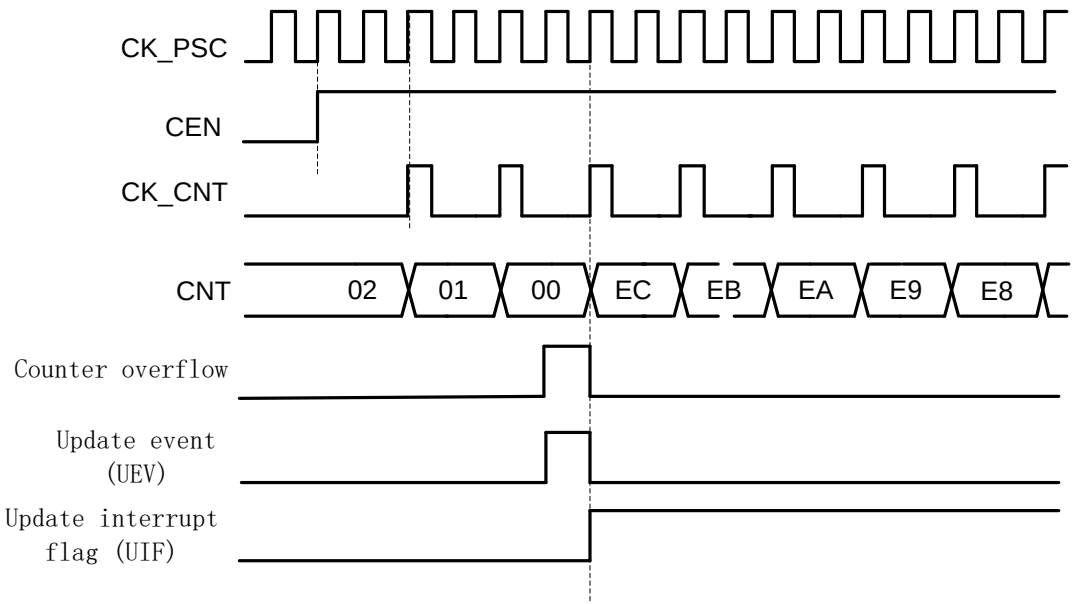
图 28-9 向下计数，内部时钟 2 分频
