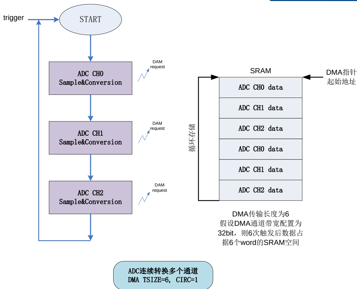
图 33-14 ADC 连续模式+DMA 循环模式
