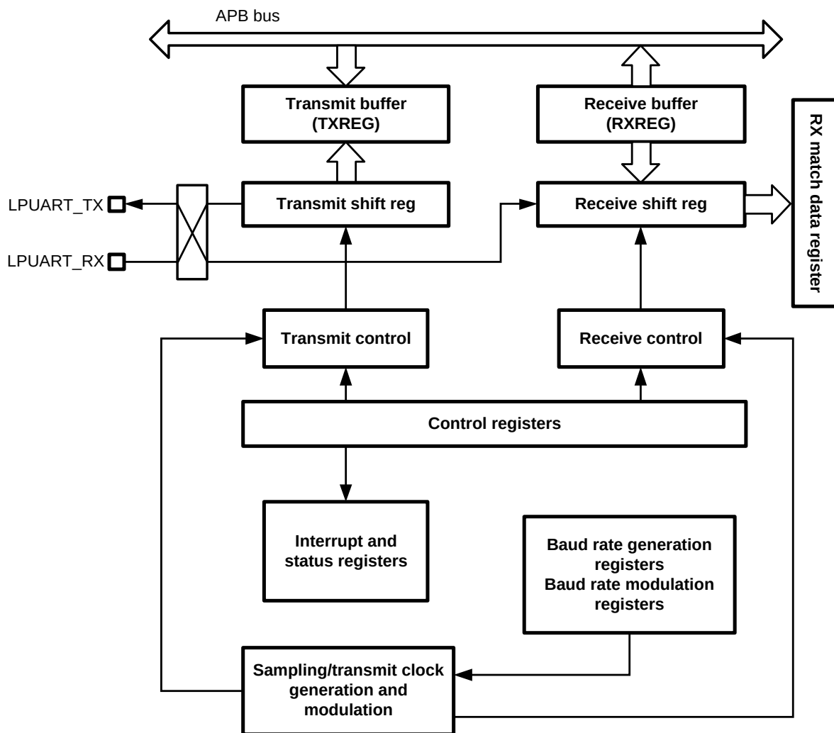
图 22-1LPUART 结构框图
