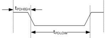
图 7.3 单总线时序图
