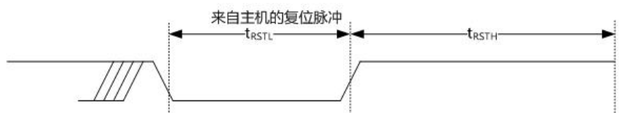
单总线存在检测
