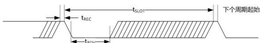
单总线复位脉冲
