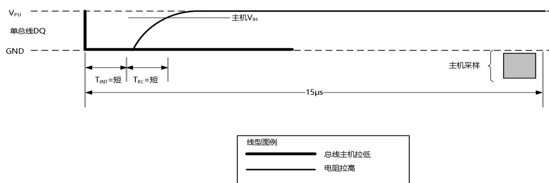
图 9.2-4 推荐的主机读 1 时序
