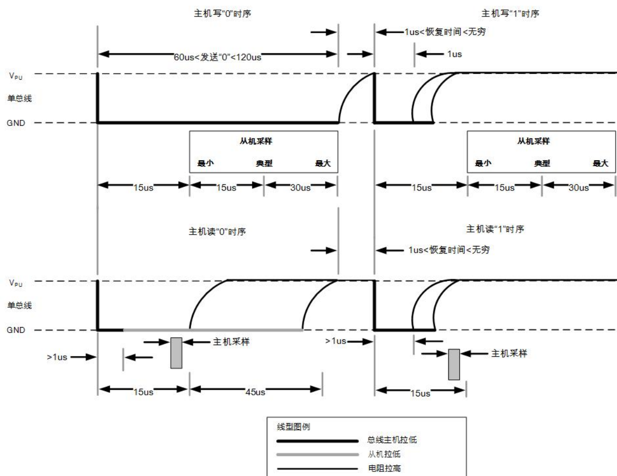
图 9.2-2 读/写时序
