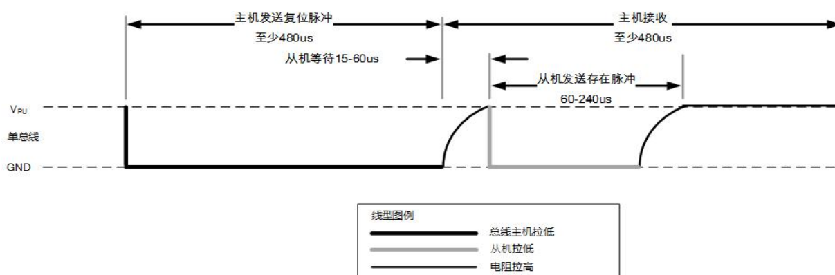
图 9.2-1 初始化时序
