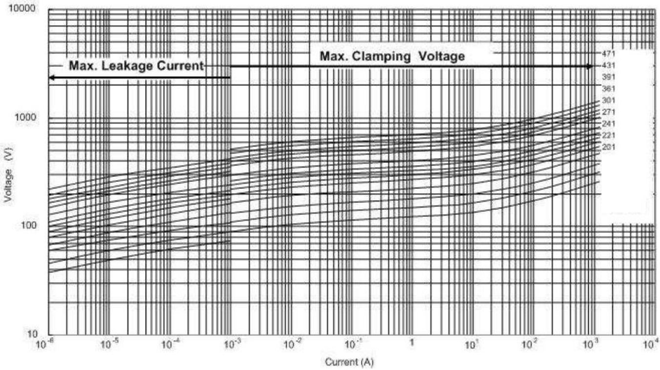
■ 最大漏电流与最大限制电压曲线 7S201K – 7S471K
