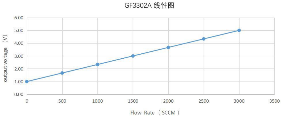
图 3. 模拟输出特性曲线（供电电压 12V）
