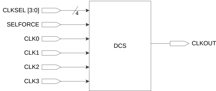
图 3-37 DCS 接口示意图
