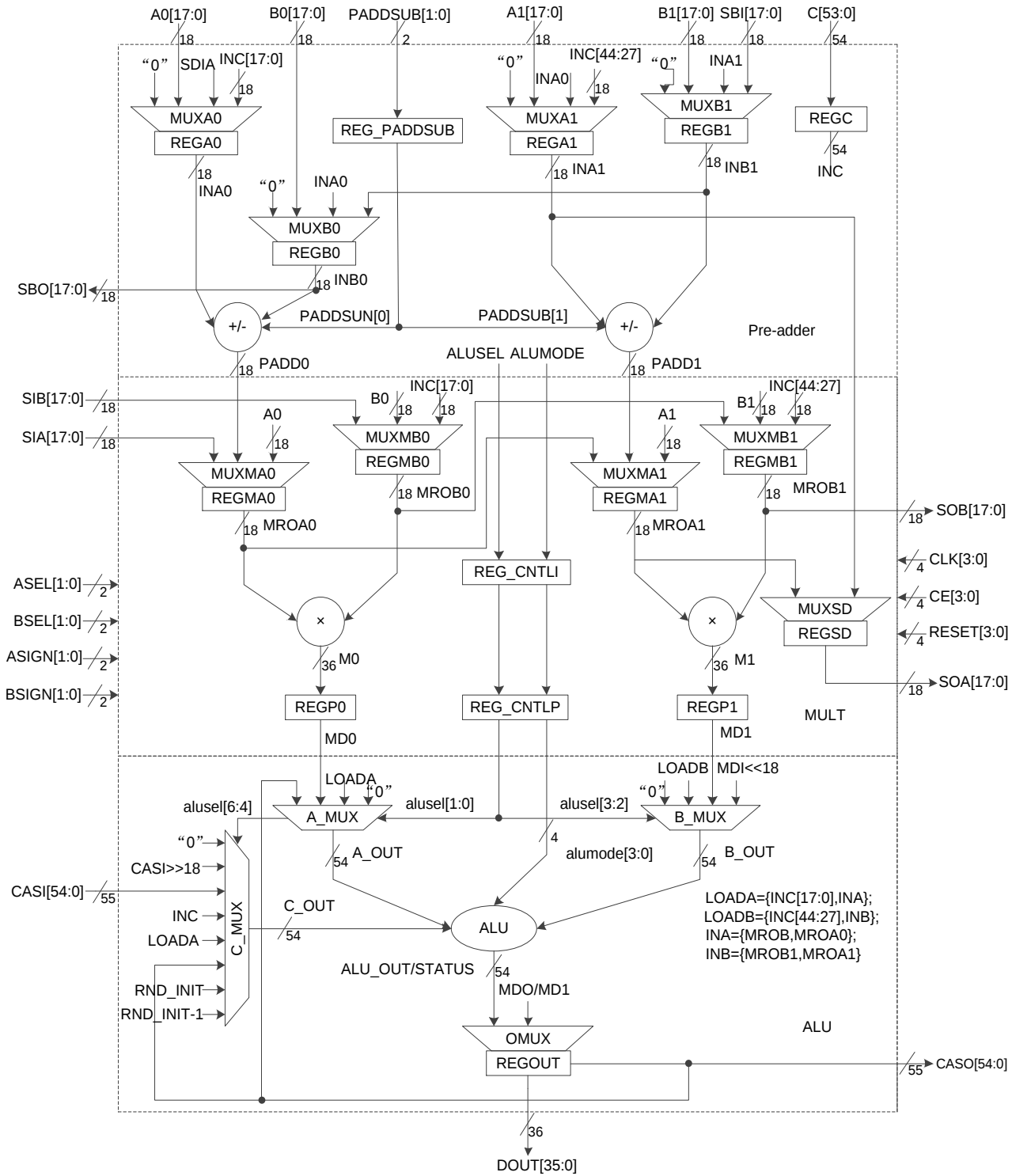
图 3-33 DSP 宏单元
