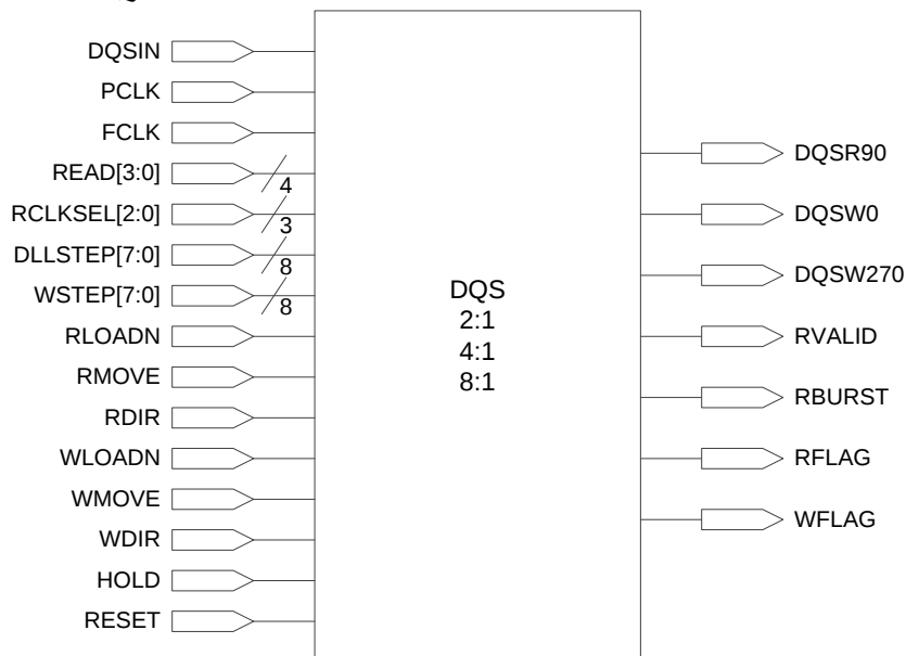
图 3-42 DQS 示意图
