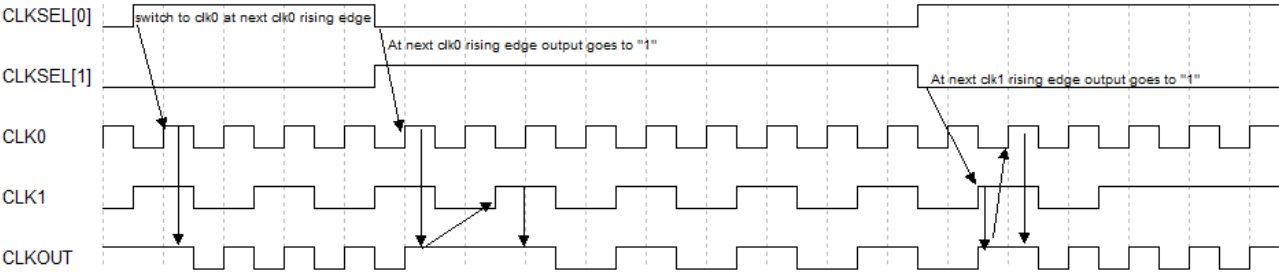
图 3-38 DCS Rising Edge 模式下的时序示意图
