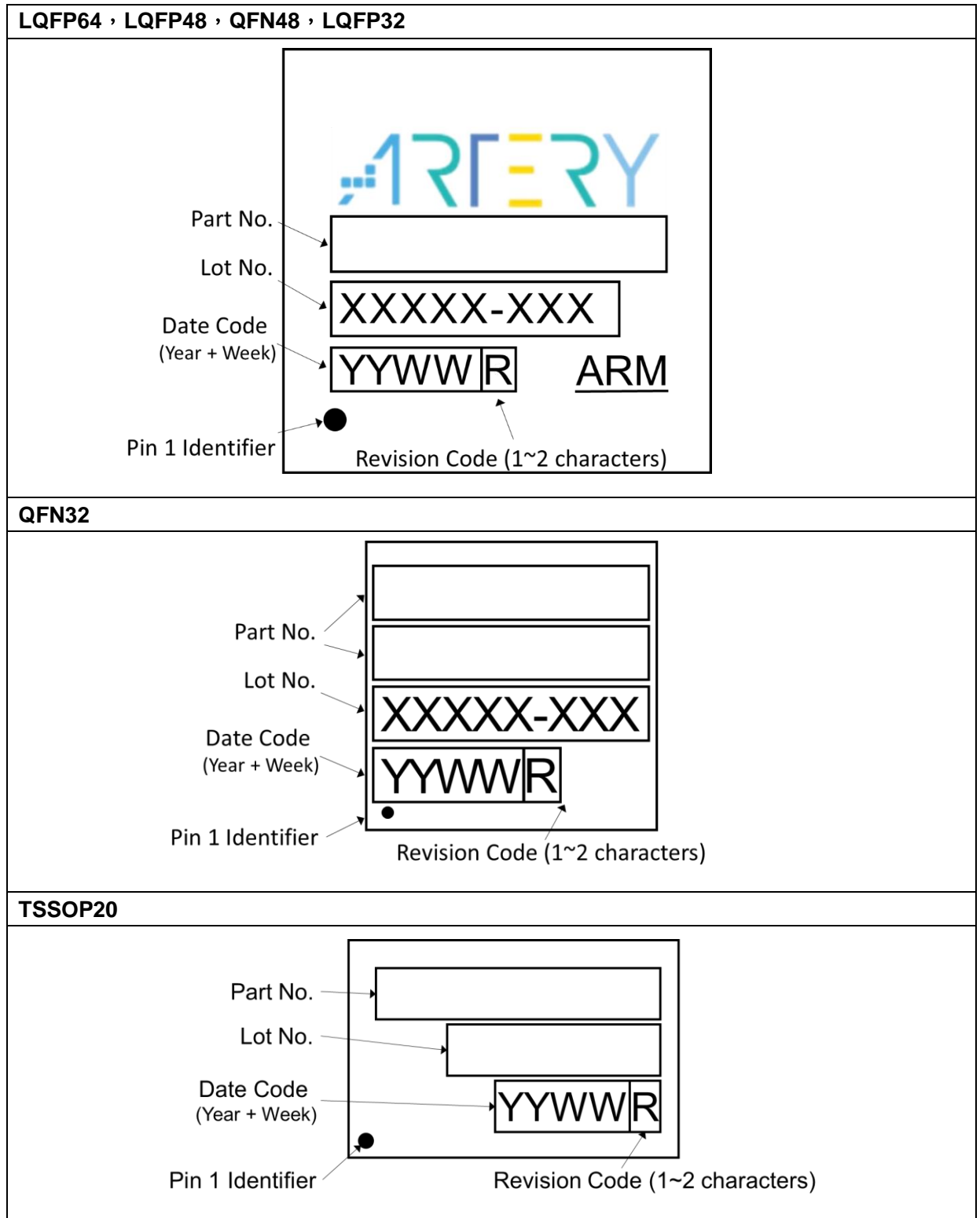
图 35. 丝印示意图
