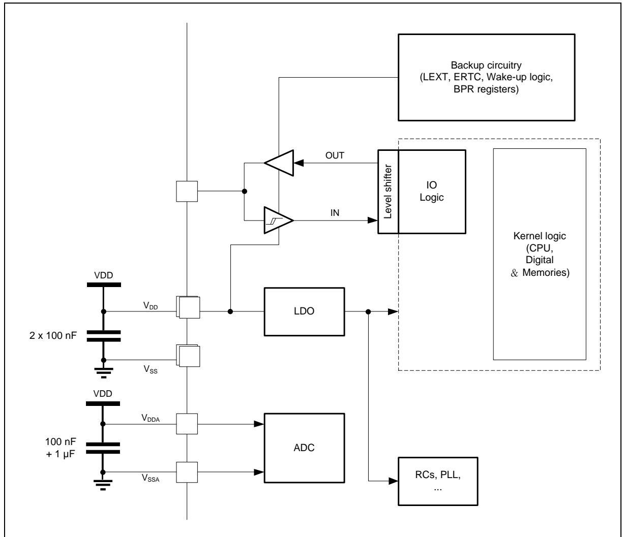
图 9. 供电方案
