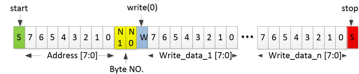
图 5.4 OWI 写操作
