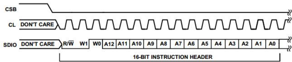
图 5.9 指令位域
