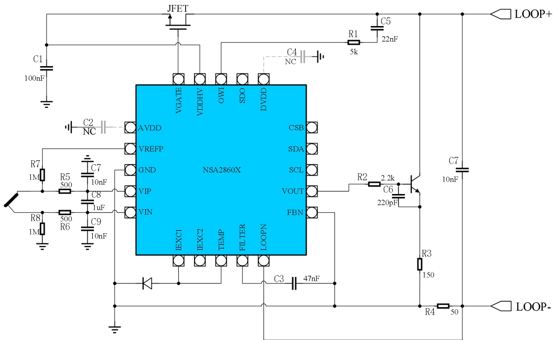
图 7.6 热电偶 4~20mA 输出温度变送器
