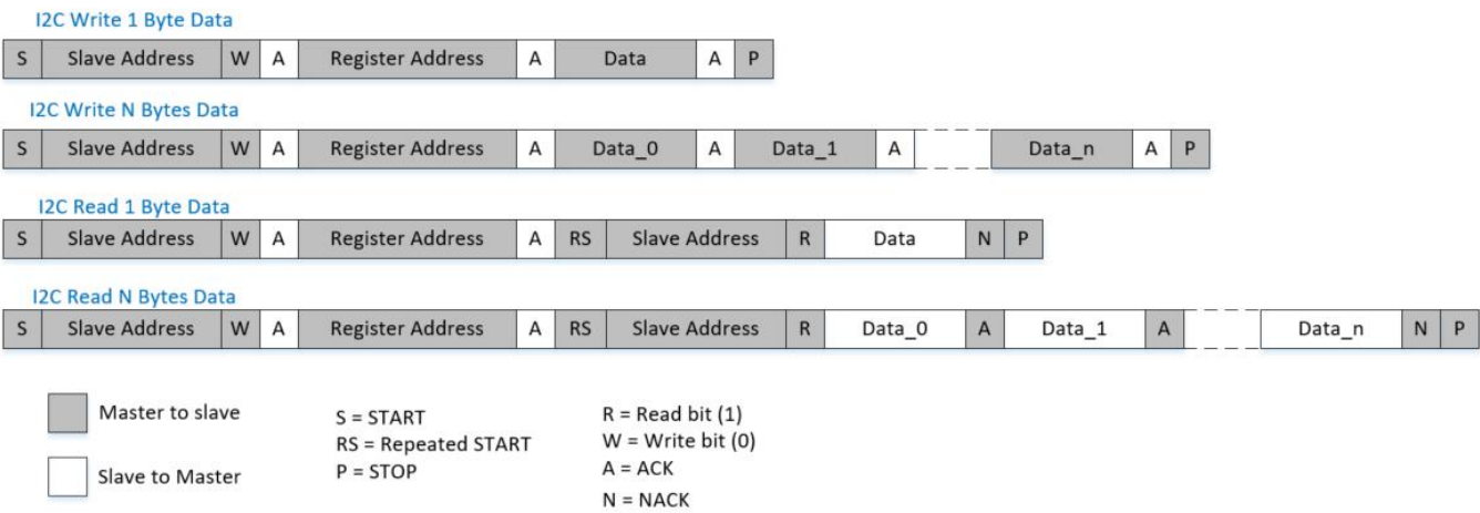
图 5.13 I2C 通讯格式
