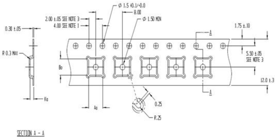
图 8.1 QFN20 编带示意图
