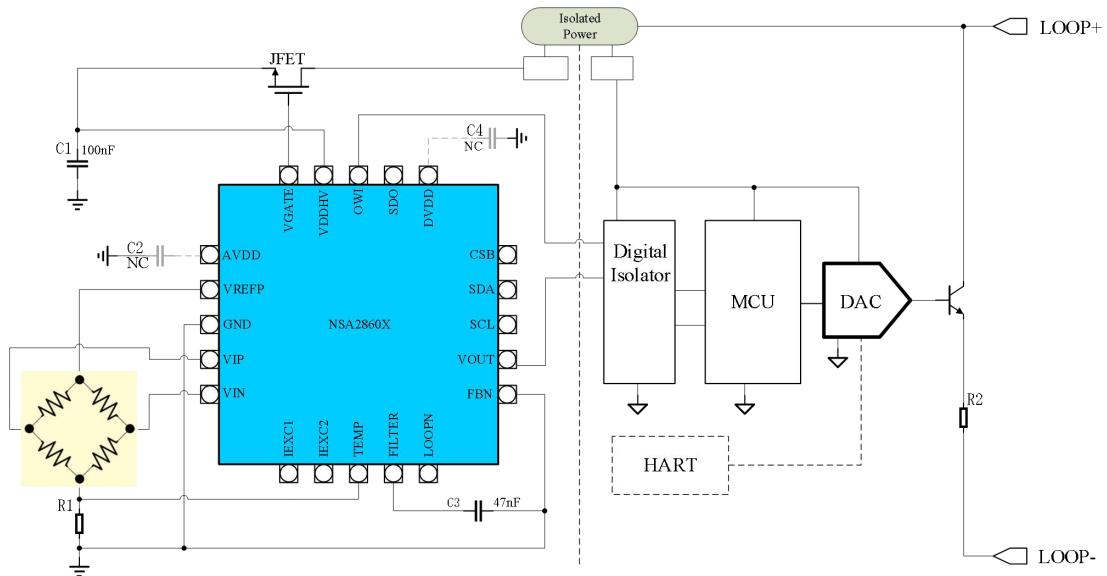
图 7.5 隔离压力变送器方案
