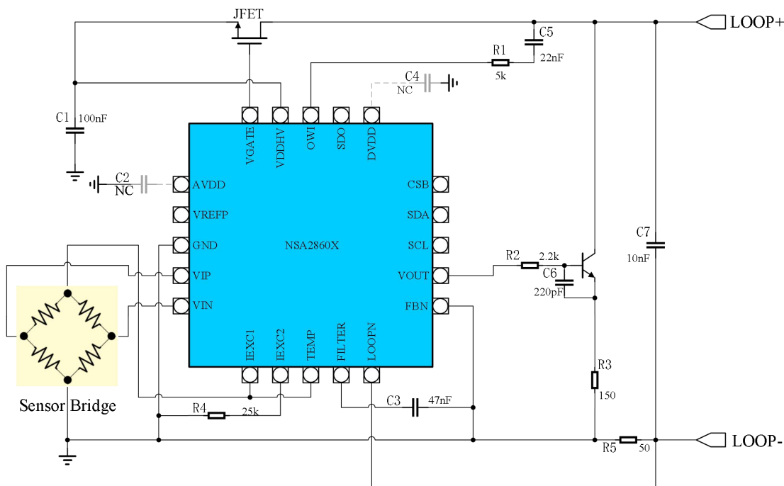
图 7.3 4~20mA 输出压力变送器(JFET)
