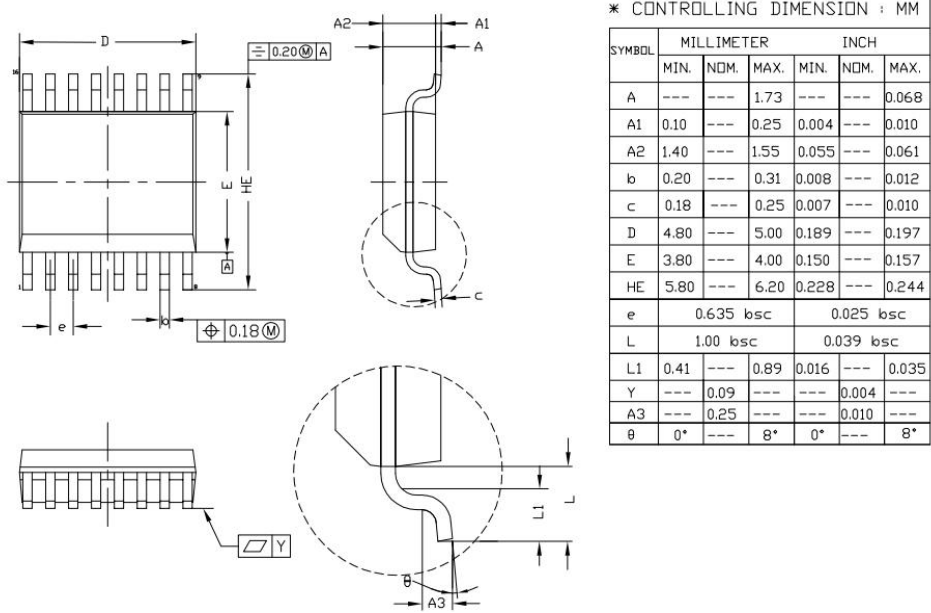
图 6.3 SSOP16 封装外形图
