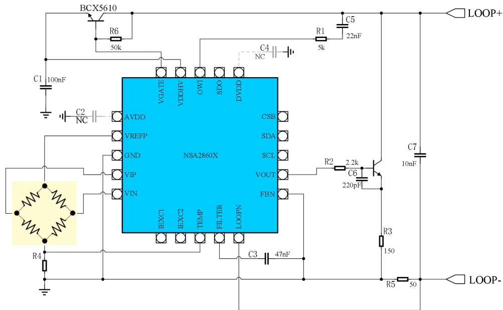
图 7.4 4~20mA 输出压力变送器(三极管)
