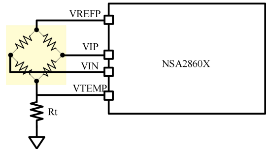
图4.3 传感器电桥和参考电阻分压作为外部温度传感器
