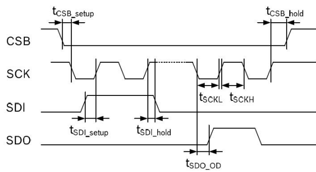
图 5.8 SPI 时序图
