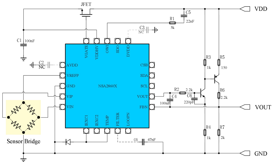
图 7.2 0~10V 输出压力变送器
