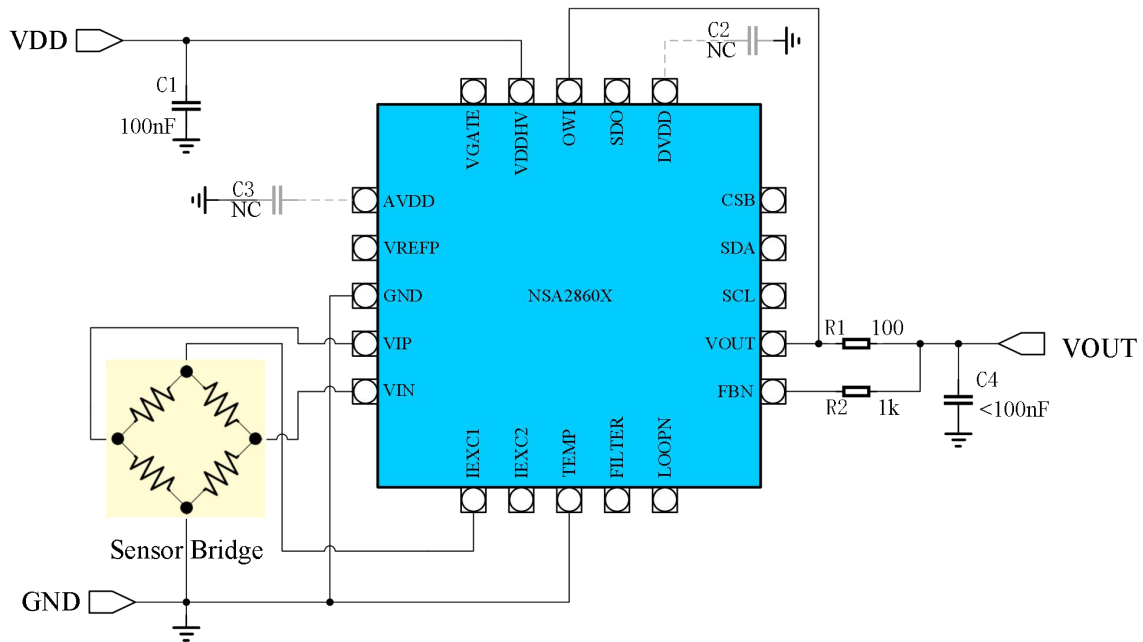
图 7.1 绝对/比例电压输出
