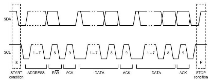
图 5.12 I2C 协议
