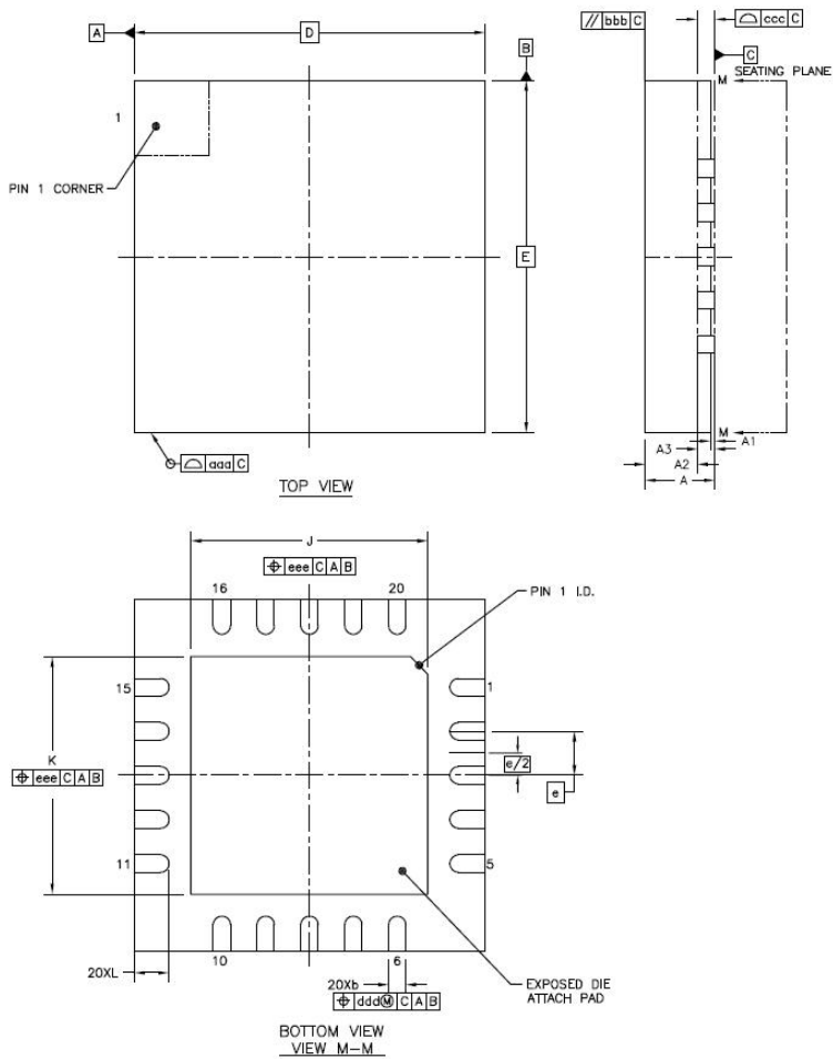
图 6.2 QFN20 封装外形图
