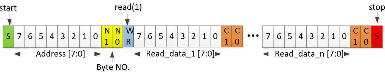
图 5.5 OWI 读操作
