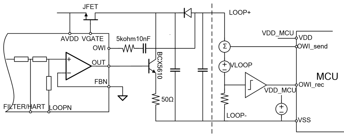
图 5.74~20mA 电流输出模式下双引脚 OWI 通讯典型连接图
