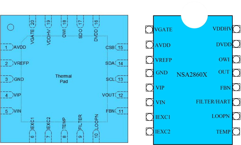
图 6.1 QFN20 和 SSOP16 封装引脚分布
