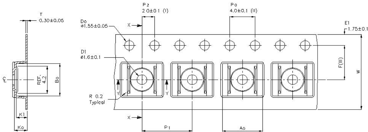
图 8.2 SSOP16 编带示意图
