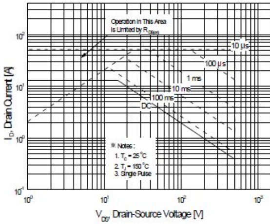
图 6-1 SIF13N50C(TO-220)
