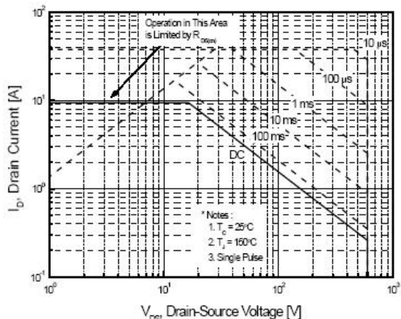
图 6-1 SIF10N60E(TO-220FP(L))
