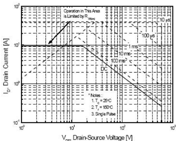
图 6-3 SIF10N60E(TO-262&263)
