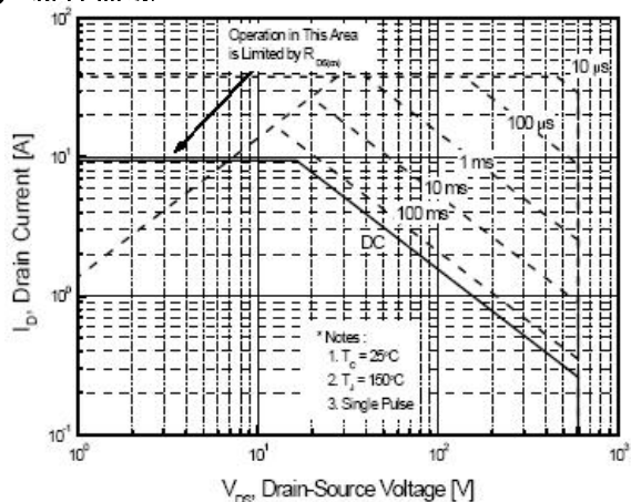
图 6-1 SIF10N60E(TO-220)
