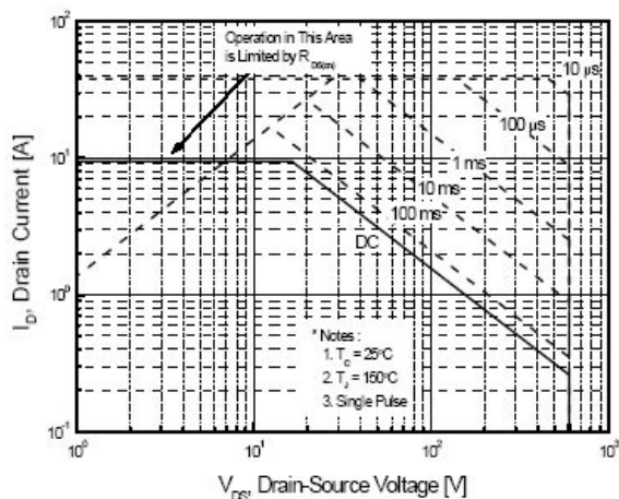
图 6-1 SIF10N65E(TO-220FP(L))
