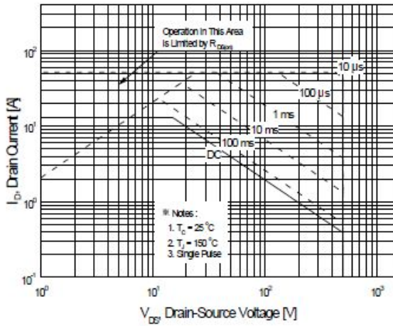
图 6-1 SIF11N50E(TO-220)
