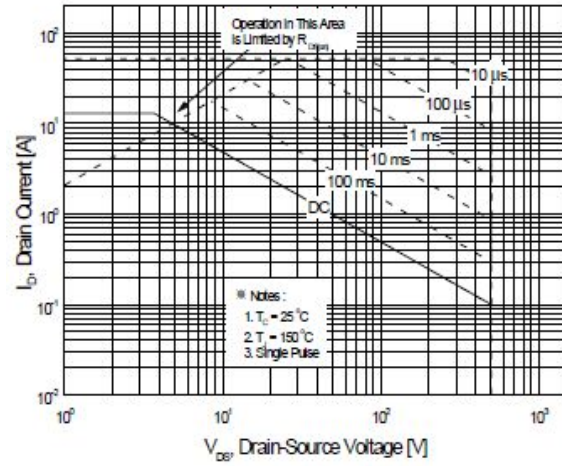
图 6-2 SIF11N50E(TO-220FP(L))
