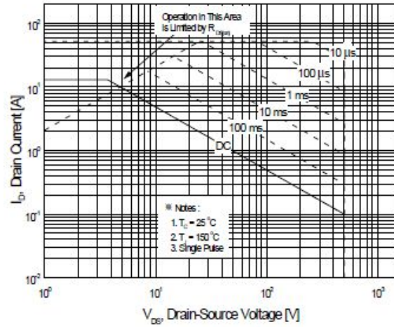
图 6-2 SIF13N50F(TO-220FP(L))
