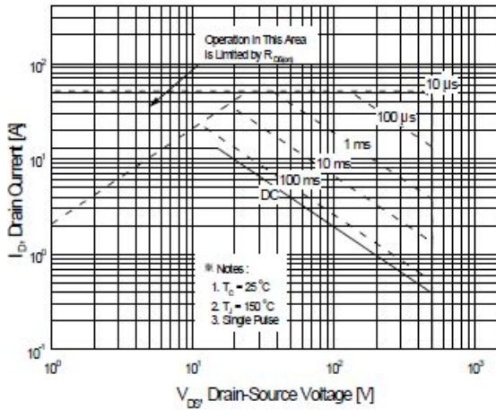
图 6-1 SIF13N50F(TO-220)
