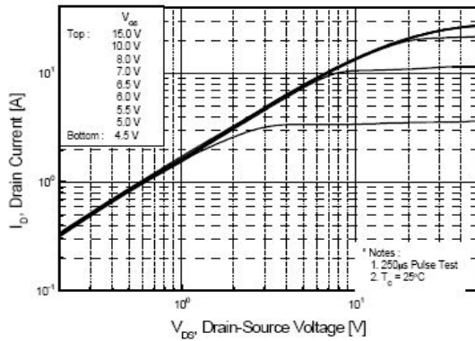
图 1 输出特性曲线, Tc=25°C
