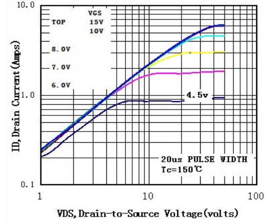
图 2 输出特性曲线, T_c=150^\circ\text{C}
