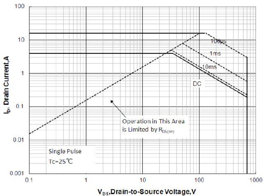
图 6-2 SIF4N70F(TO-220FP/251T/252(T))
