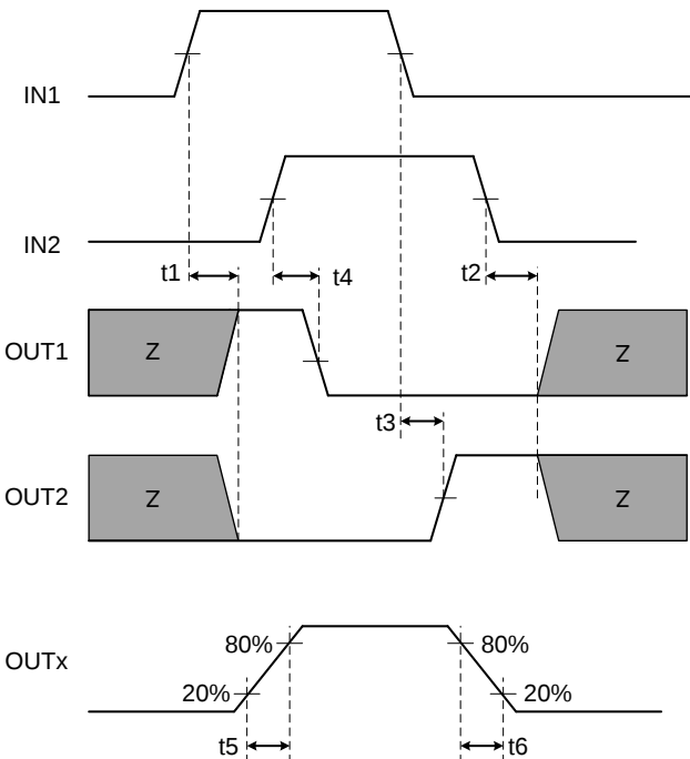
图 5. 输入输出时序图
