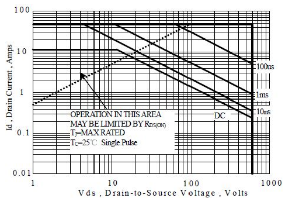
图 6-1 SIF12N60F(TO-220)
