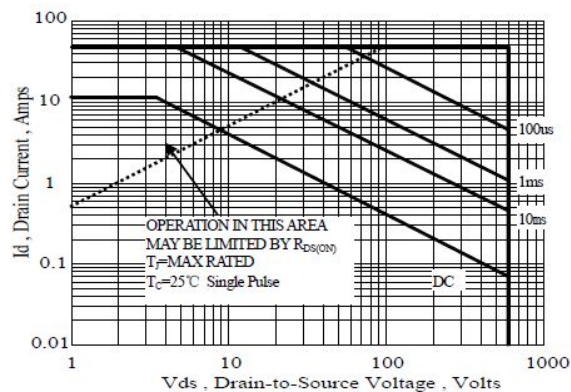
图 6-2 SIF12N60F(TO-220FP(L))
