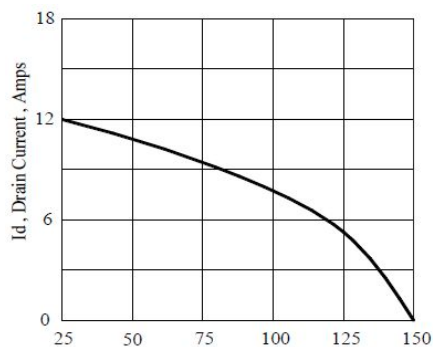
图 5 最大漏极电流与壳温曲线
