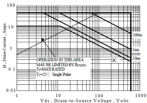
图 6-3 SIF12N60F(TO-262&263)
