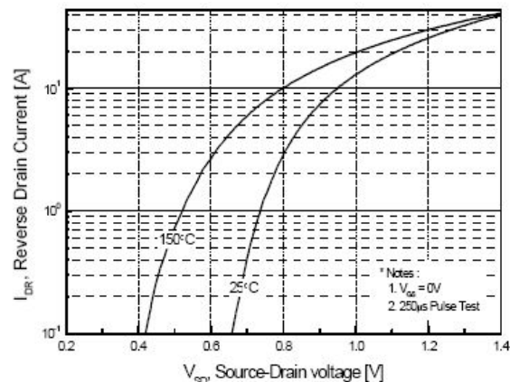
图 4 二极管正向压降曲线
