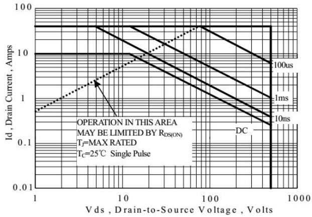
图 6-1 SIF10N50F(TO-220)
