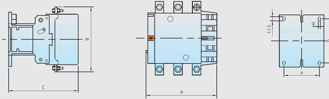
NC7-410~475
