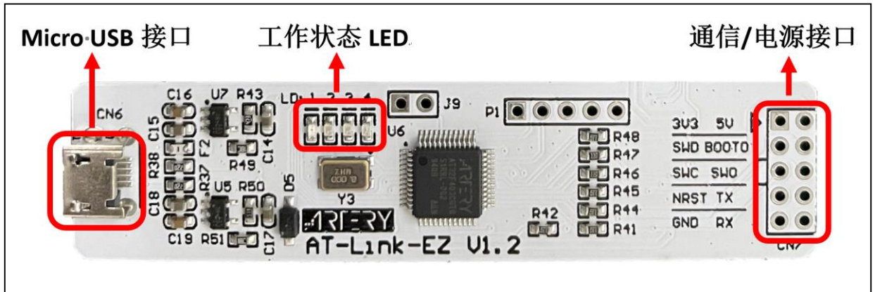
图 2. AT-Link-EZ 硬件外观接口
