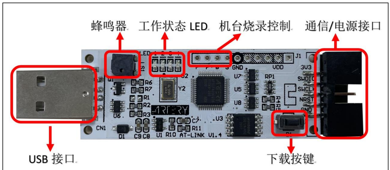
图 1. AT-Link 硬件外观接口
