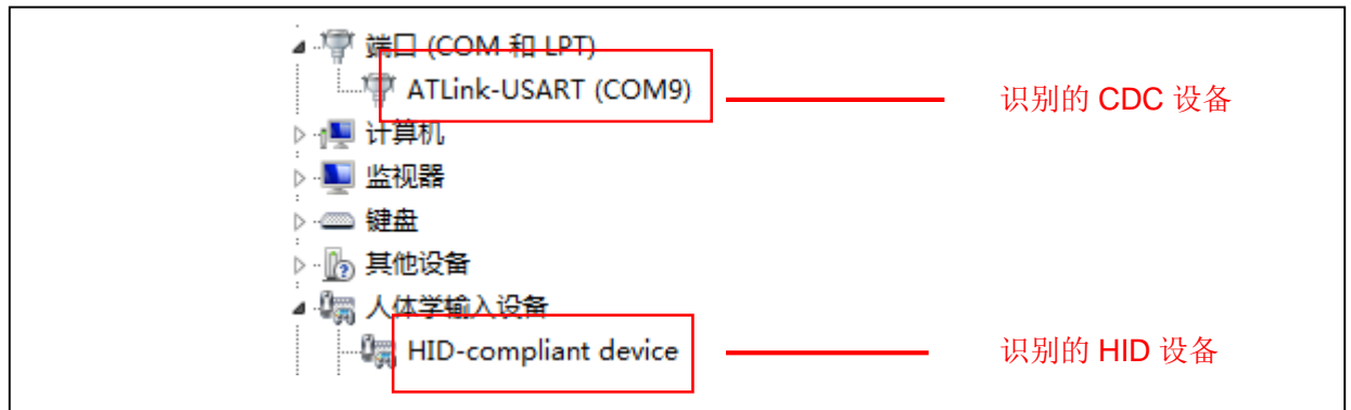
图 6. WIN7 系统设备管理器识别
