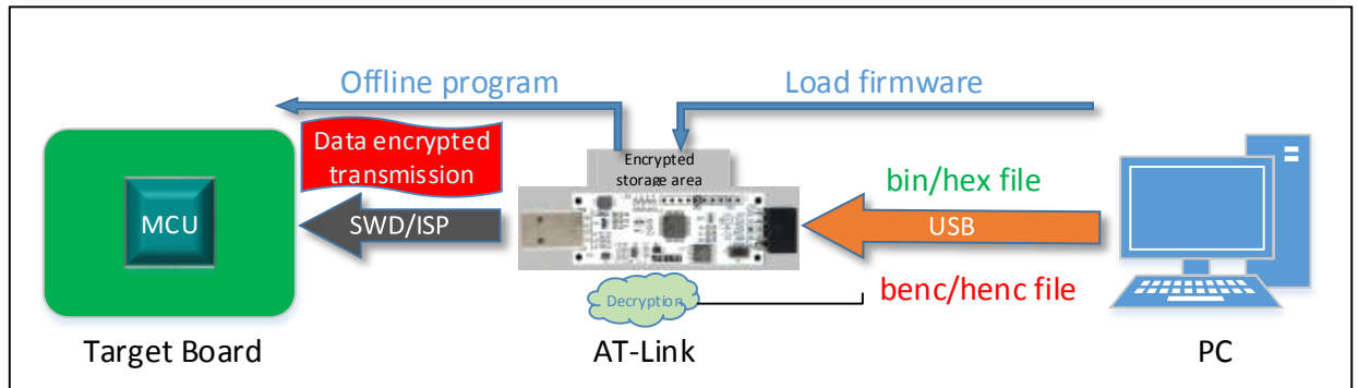
图 21. 离线编程流程图
