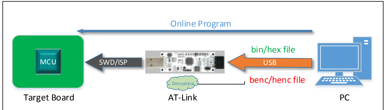
图 18. 在线编程流程图
