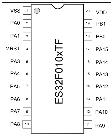
图 3-1 ES32F0100TF TSSOP20 顶视图
