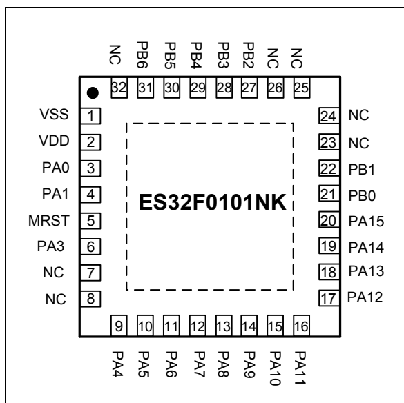
图 3-2 ES32F0101NK QFN32 顶视图
