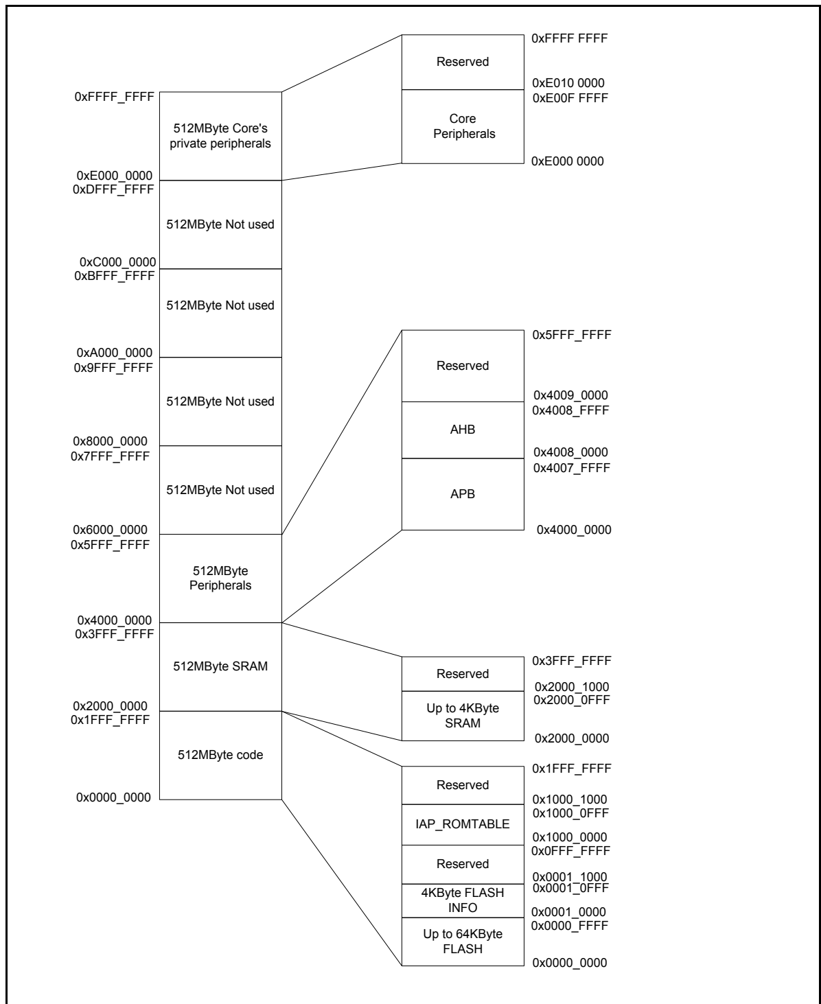
图 4-1 存储器映射
