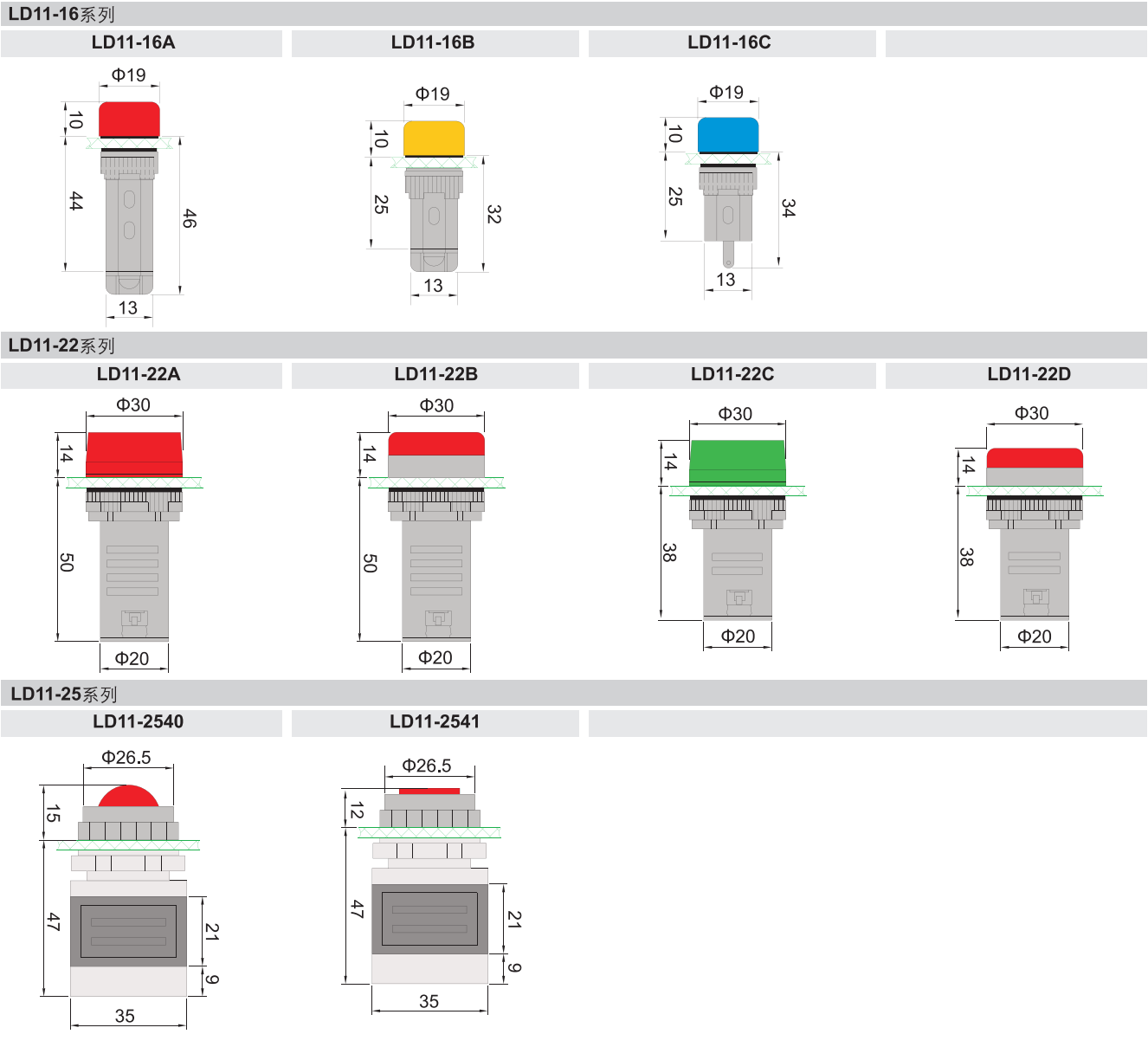
外形及安装尺寸(mm)
