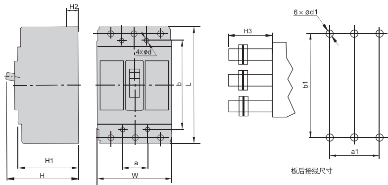
外形及安装尺寸(mm)
