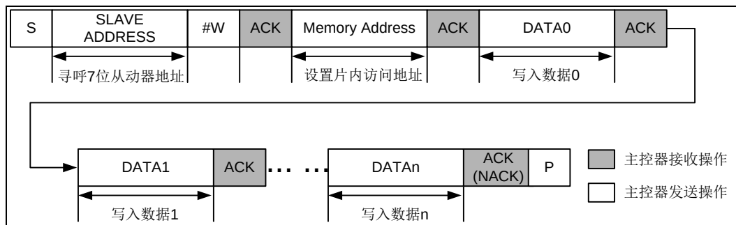
图 6-48 主控制器写入从动器数据示意图
