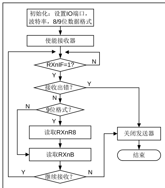
图 6-40 UARTn 接收器操作流程图
