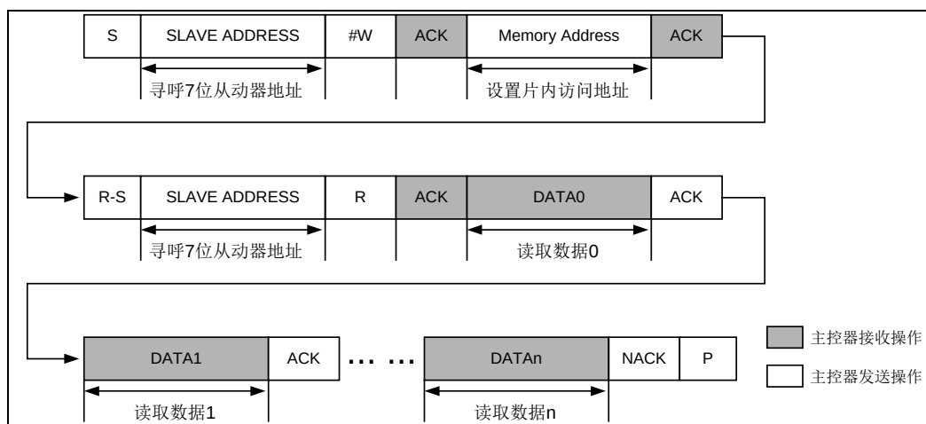
图 6-49 主控制器读取从动器数据示意图
