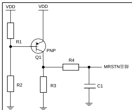
图 5-8 MRSTN 复位参考电路图 2
