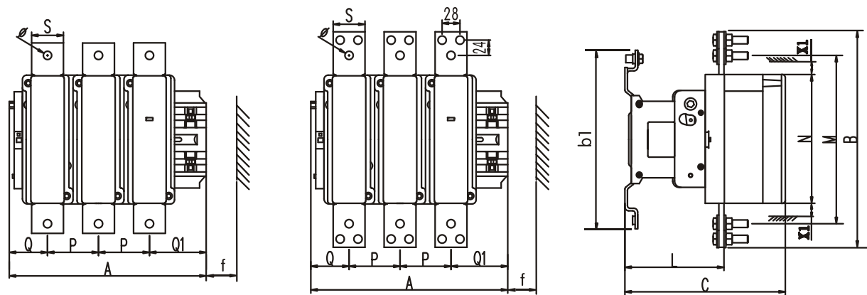
CJX2sF-1000、1250 外形
