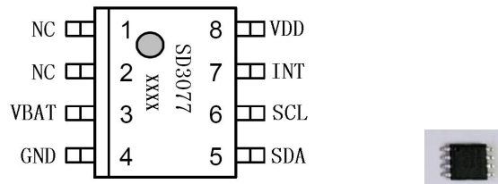
SD3077 管脚功能表
