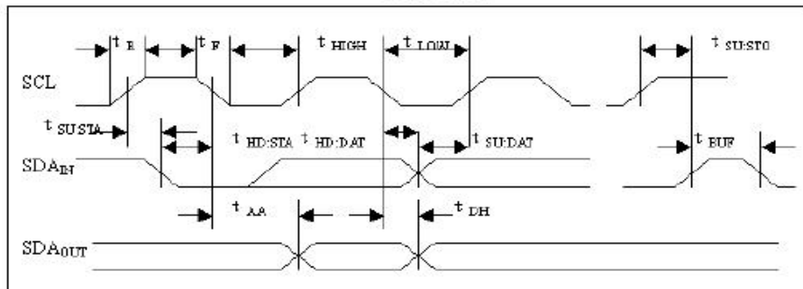
总线时序图
