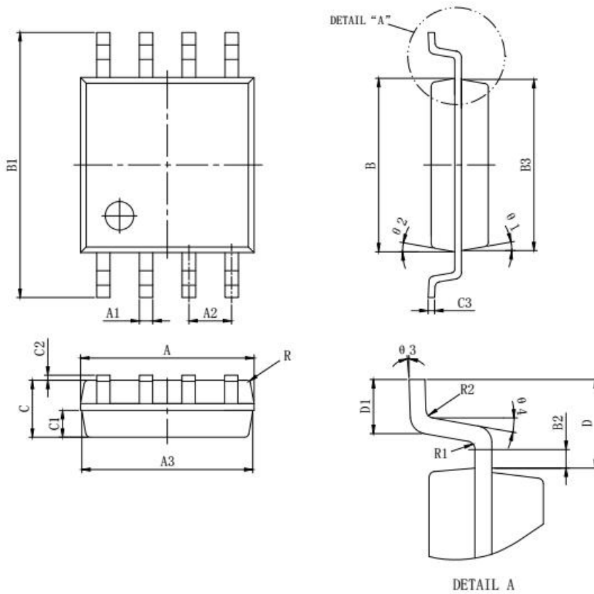
SD3077 宽体 SOP8 (208mil 宽) 封装尺寸图
