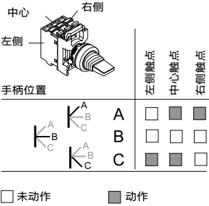
触点状态, 3位置
