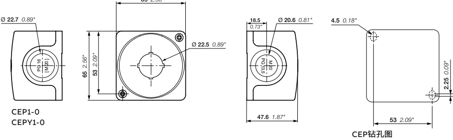
CEP钻孔图
