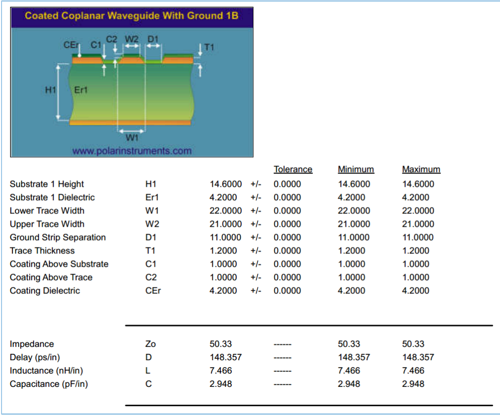
图 4-9 阻抗控制叠层设计
