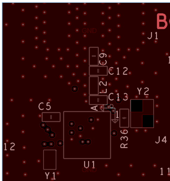
图 4-18 L2层设计
