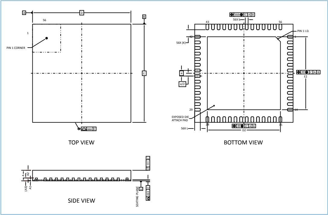
图 7-3 QFN56封装外形尺寸
