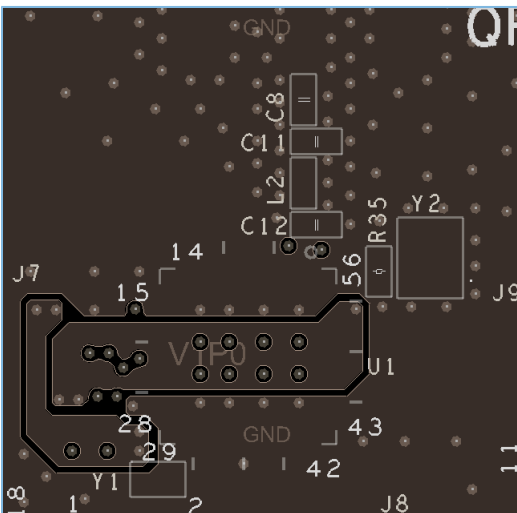
图 4-12 L3层设计
