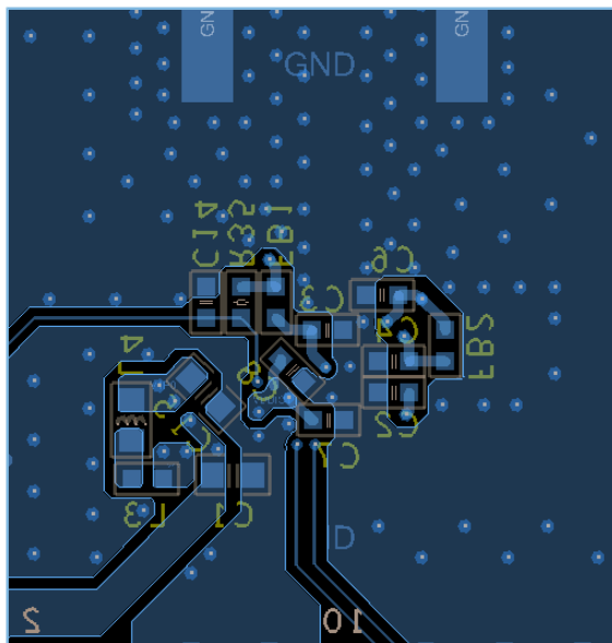
图 4-20 BOTTOM层设计
