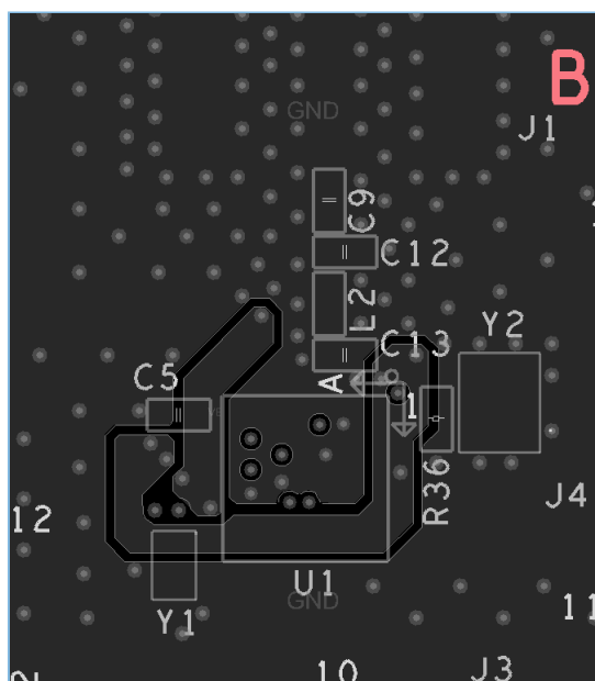
图 4-19 L3层设计
