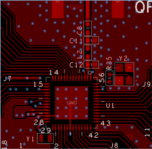
图 4-10 TOP层设计
