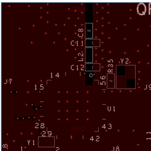
图 4-11 L2层设计
